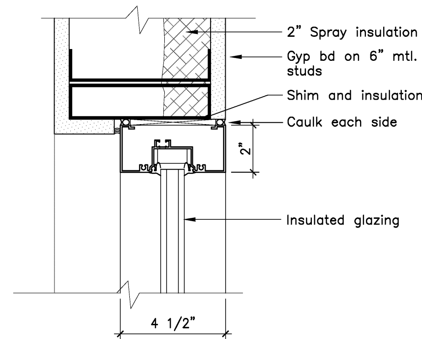
10 Storefront Head Detail Scale: 3" = 1'-0"
