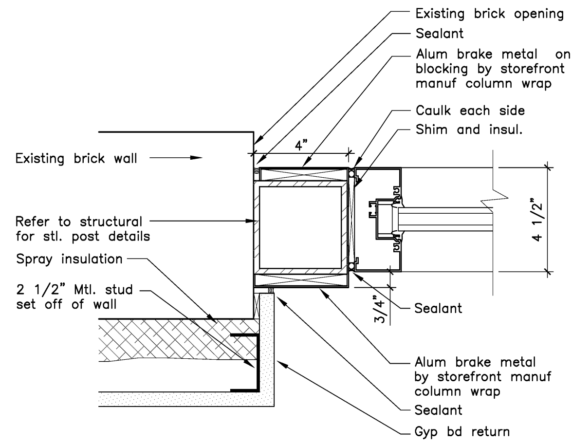
12 Storefront Jamb Detail Scale: 3" = 1'-0"
