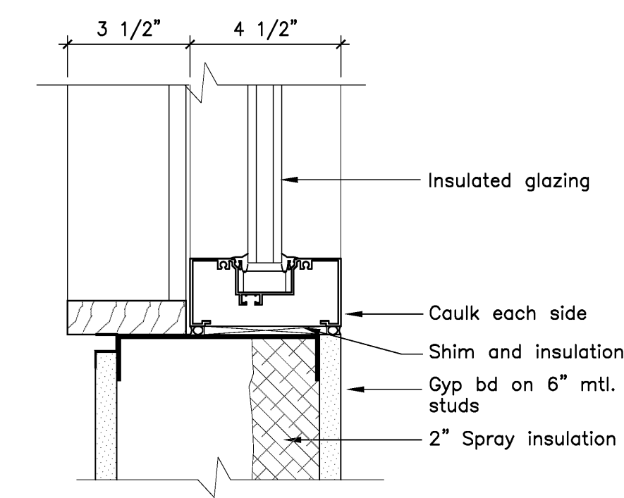
14 Storefront Jamb Detail - Alternate #3 Scale: 3" = 1'-0"
