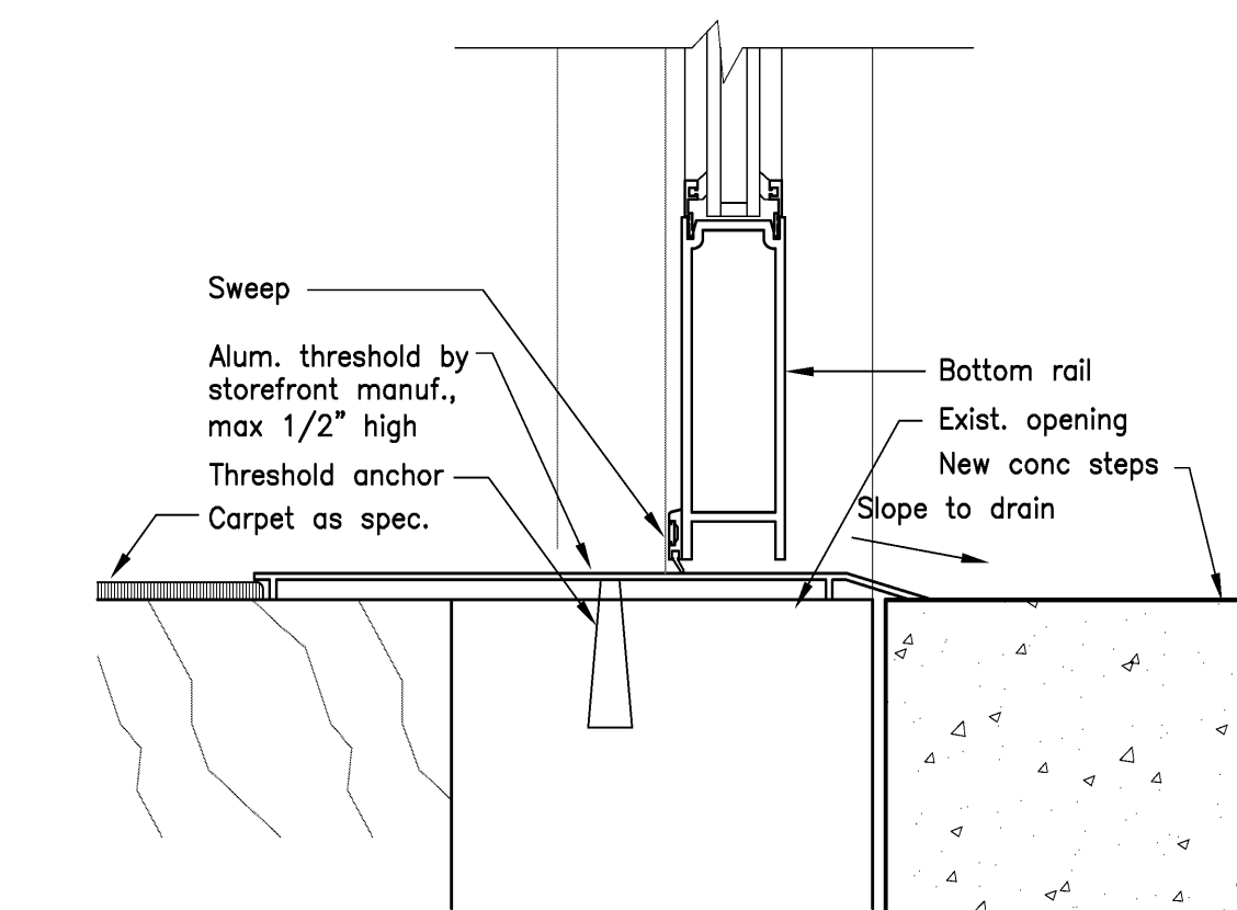
3 Storefront Entrance Scale: 3" = 1'-0"
