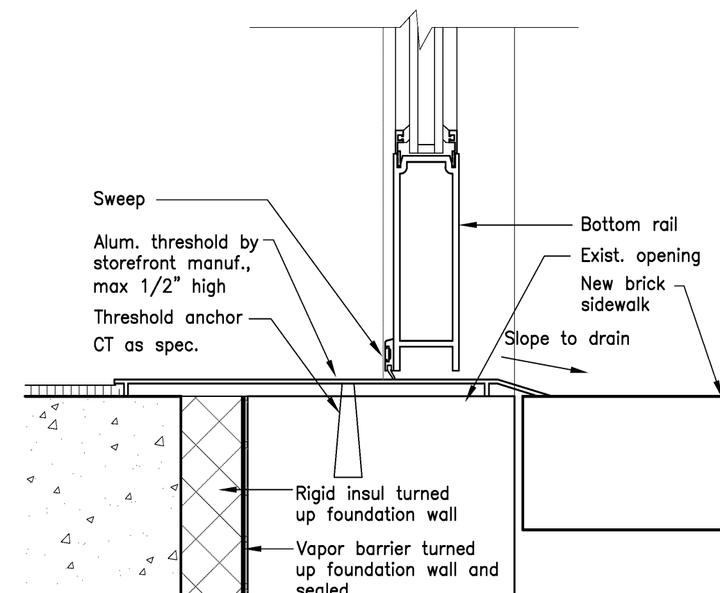
7 Storefront Entrance Scale: 3" = 1'-0"
