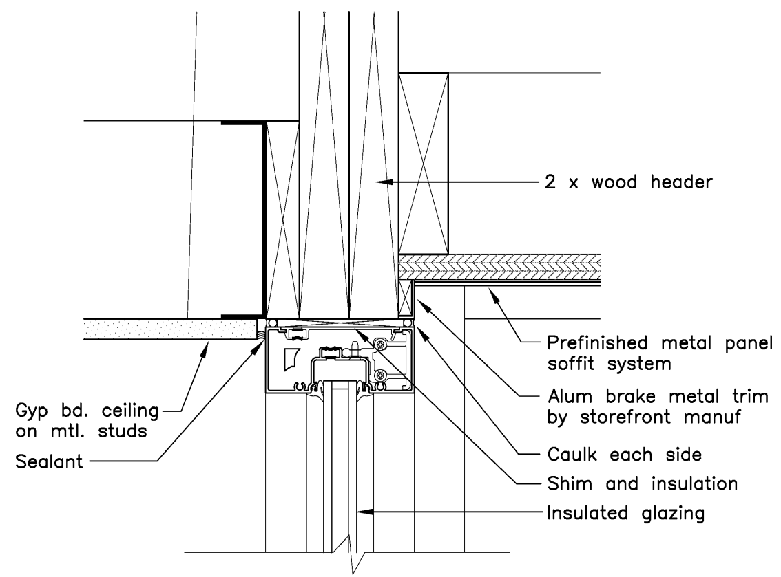
9 Storefront Head Detail Scale: 3" = 1'-0"
