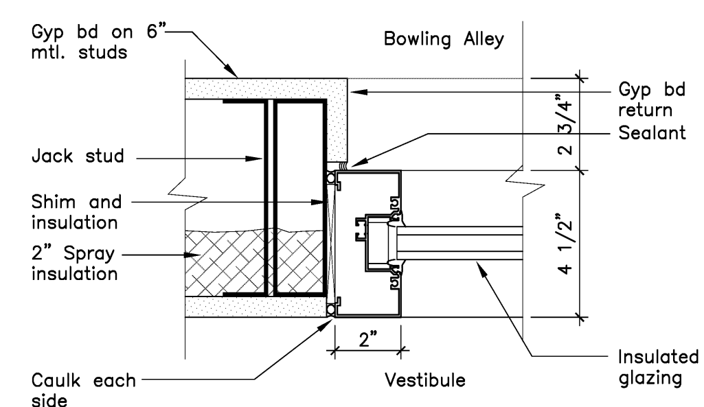
8 Storefront Jamb Detail Scale: 3" = 1'-0"
