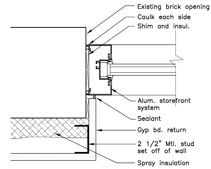
5 Storefront Jamb Detail Scale: 3" = 1'-0"
