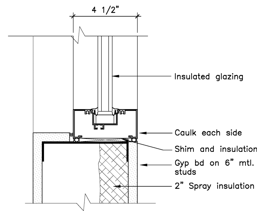
11 Storefront Jamb Detail Scale: 3" = 1'-0"
