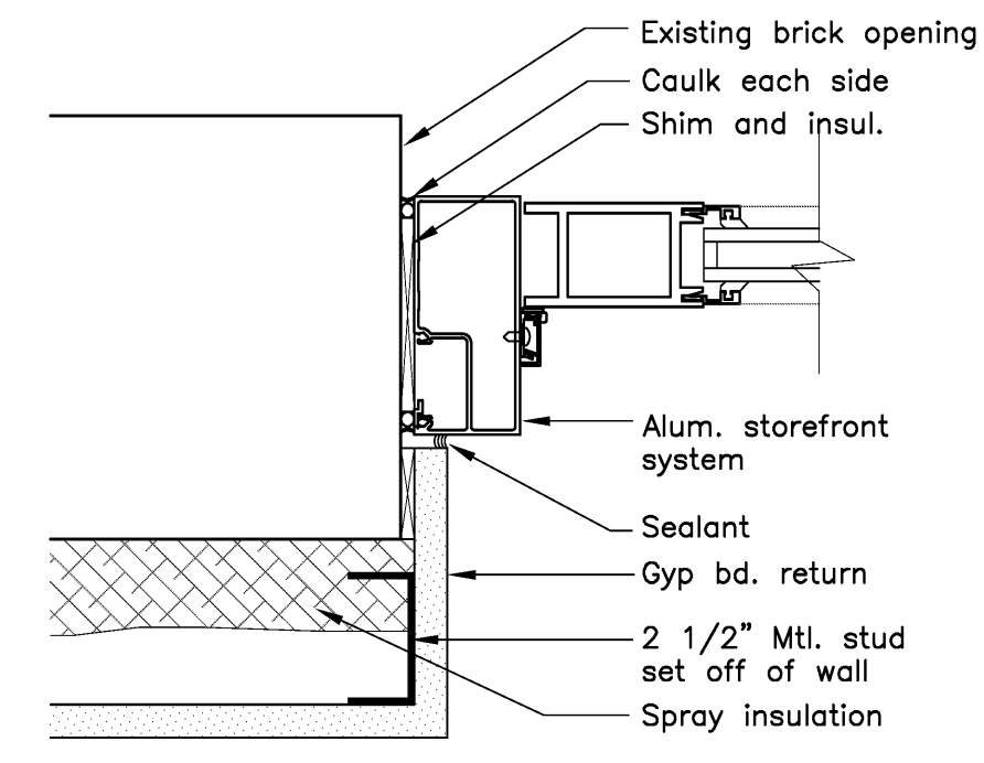
6 Storefront Jamb Detail Scale: 3" = 1'-0"
