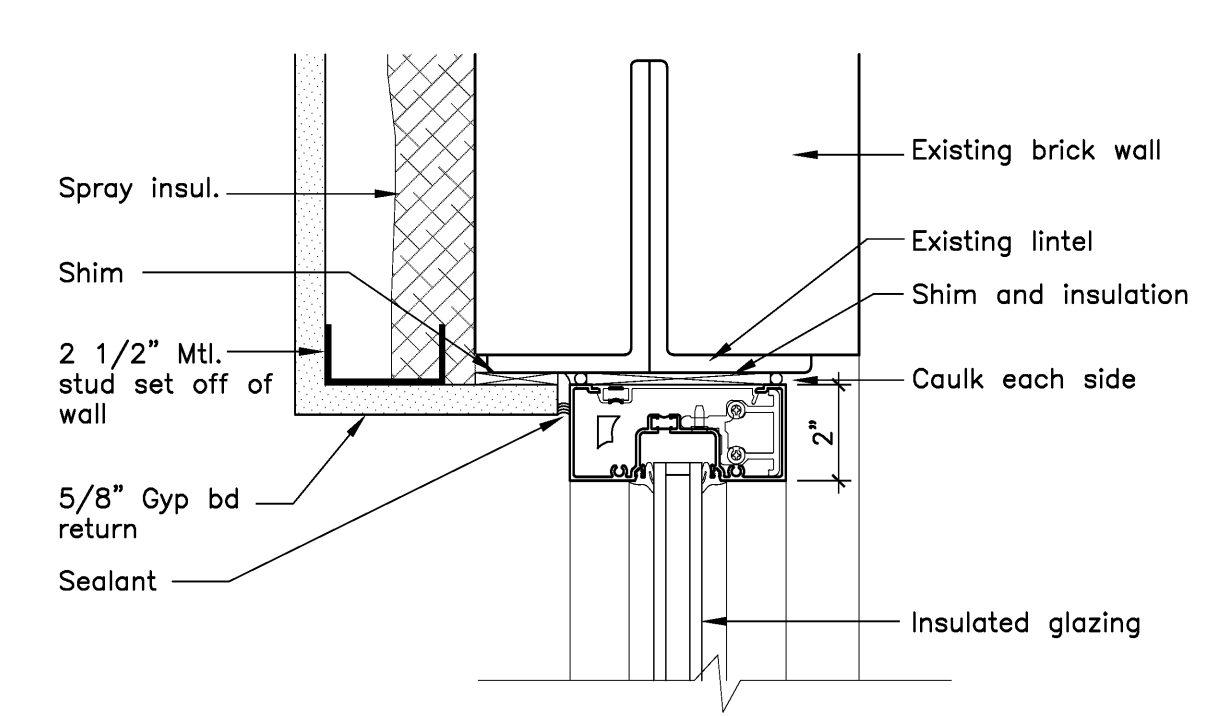
1 Storefront Head Detail Scale: 3" = 1'-0"
