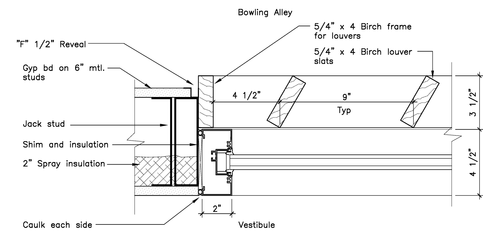
3 Storefront Entrance Scale: 3" = 1'-0"
