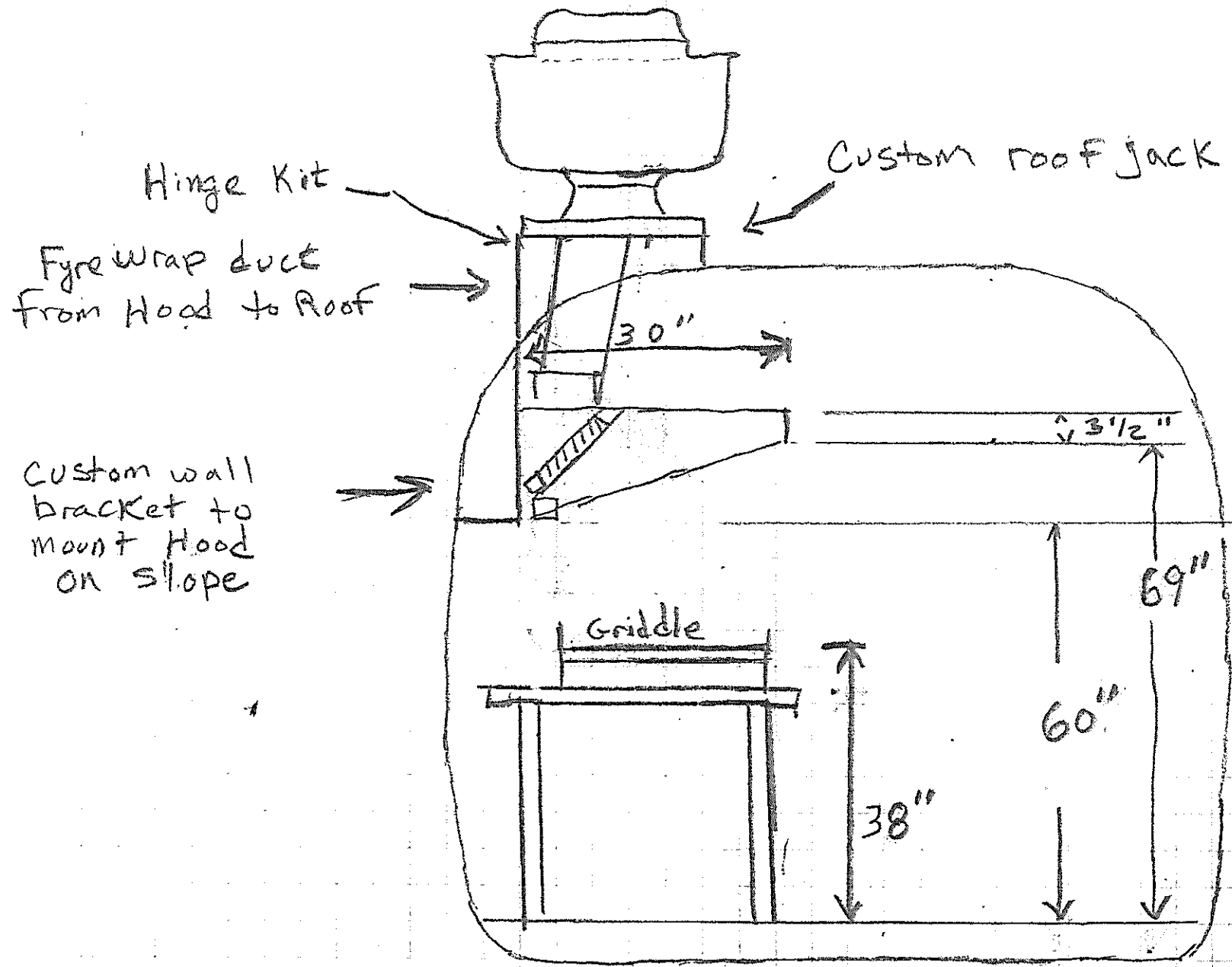
Section A-A
