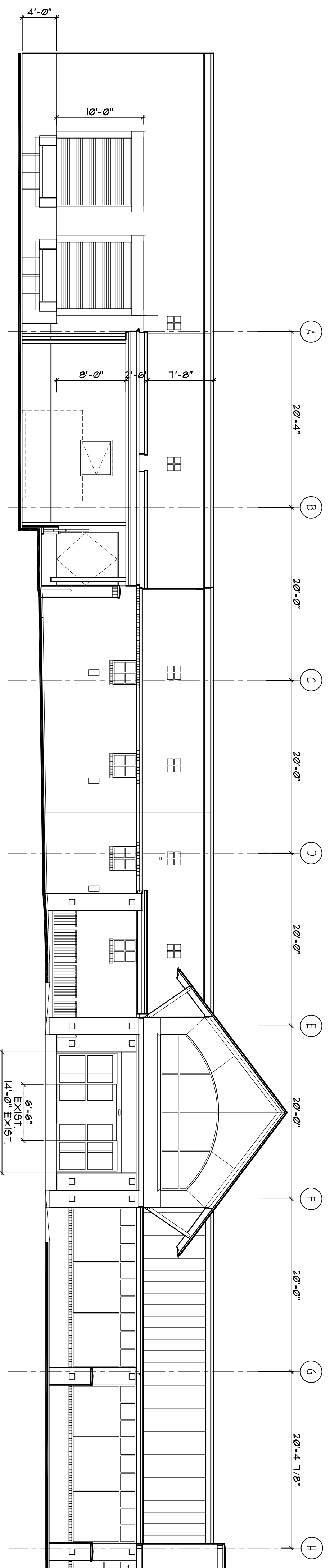
EXISTING CONDITION - STOREFRONT ELEVATION SCALE: 1/8" = 1'-0"
