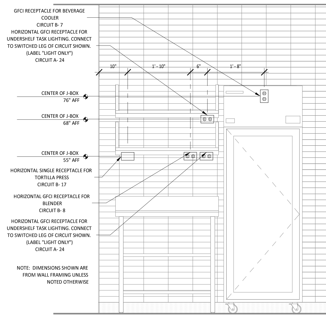
CHIP TABLE ELECTRICAL ELEVATION E300 N.T.S.
