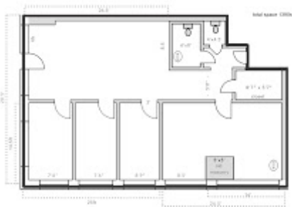
ExistingFloorPlan.jpg 1120K
