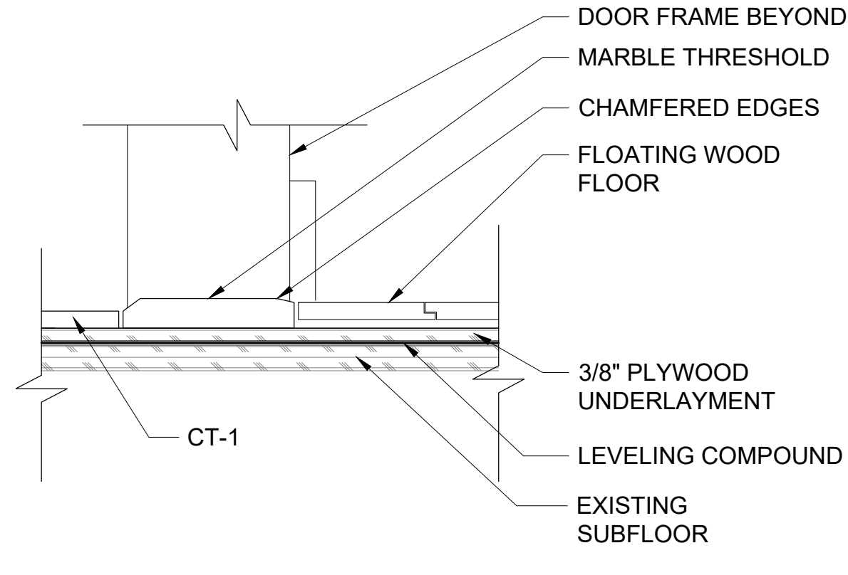
3 TILE/HARDWOOD TRANS. SCALE: 3" = 1'-0"
