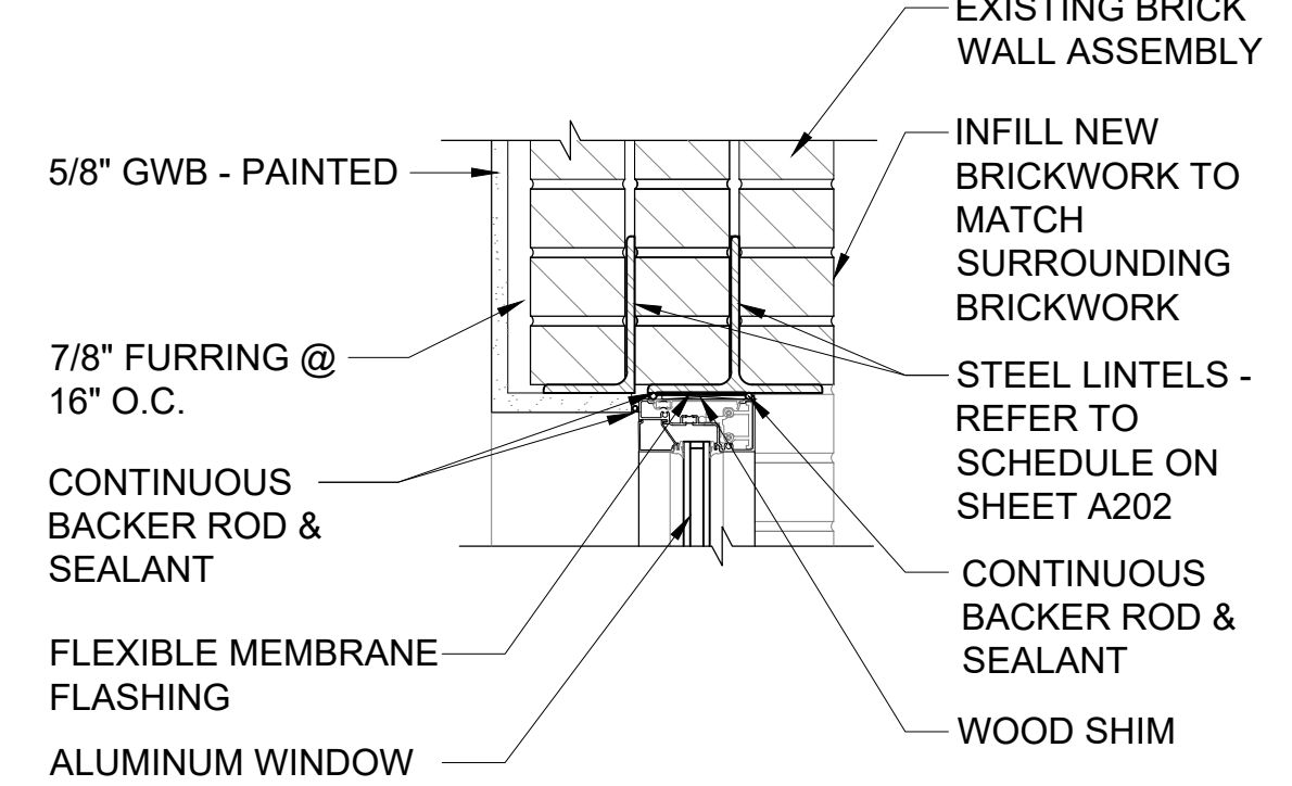
13 WINDOW "J" HEAD SCALE: 1-1/2" = 1'-0"
