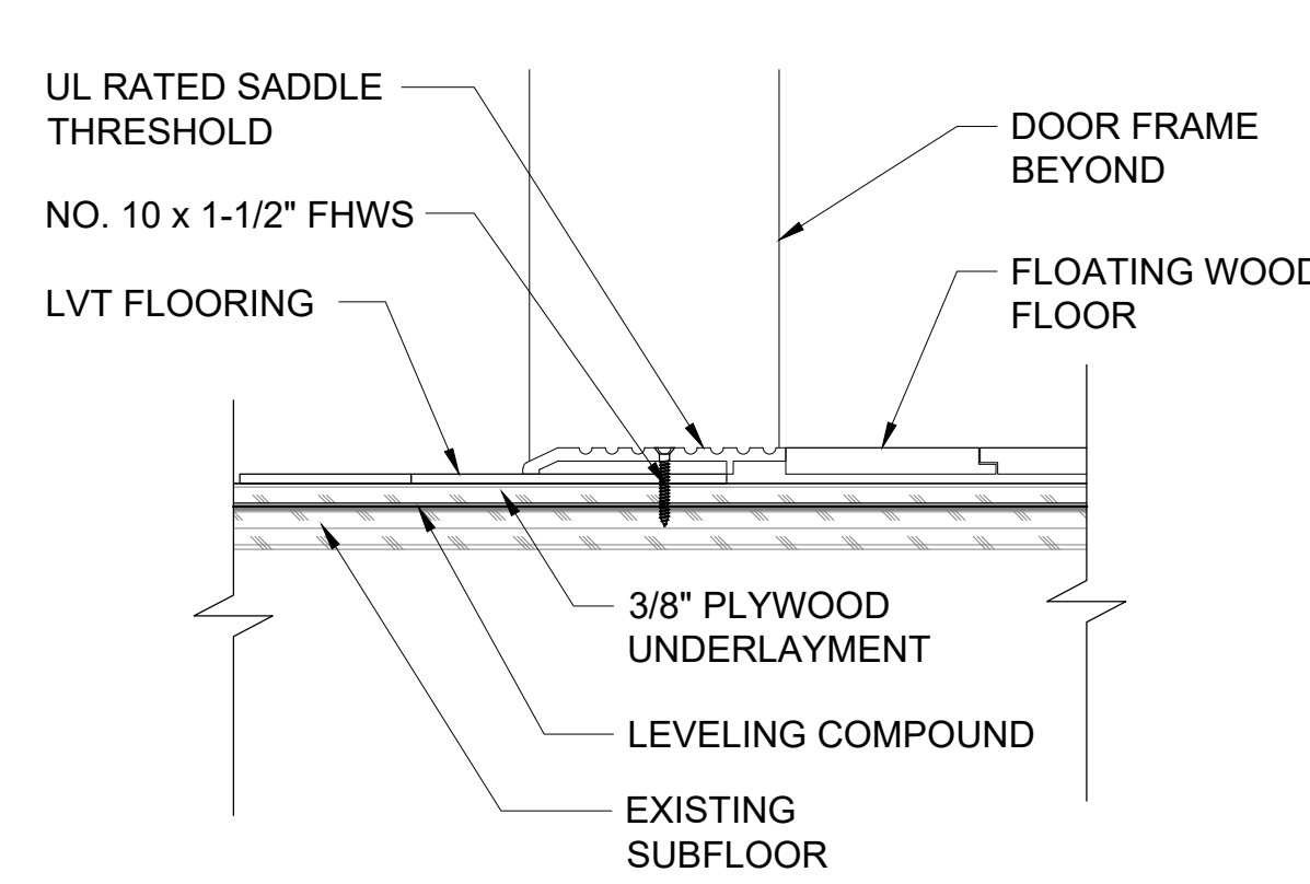
4 APT ENTRY DOOR SILL SCALE: 3" = 1'-0"
