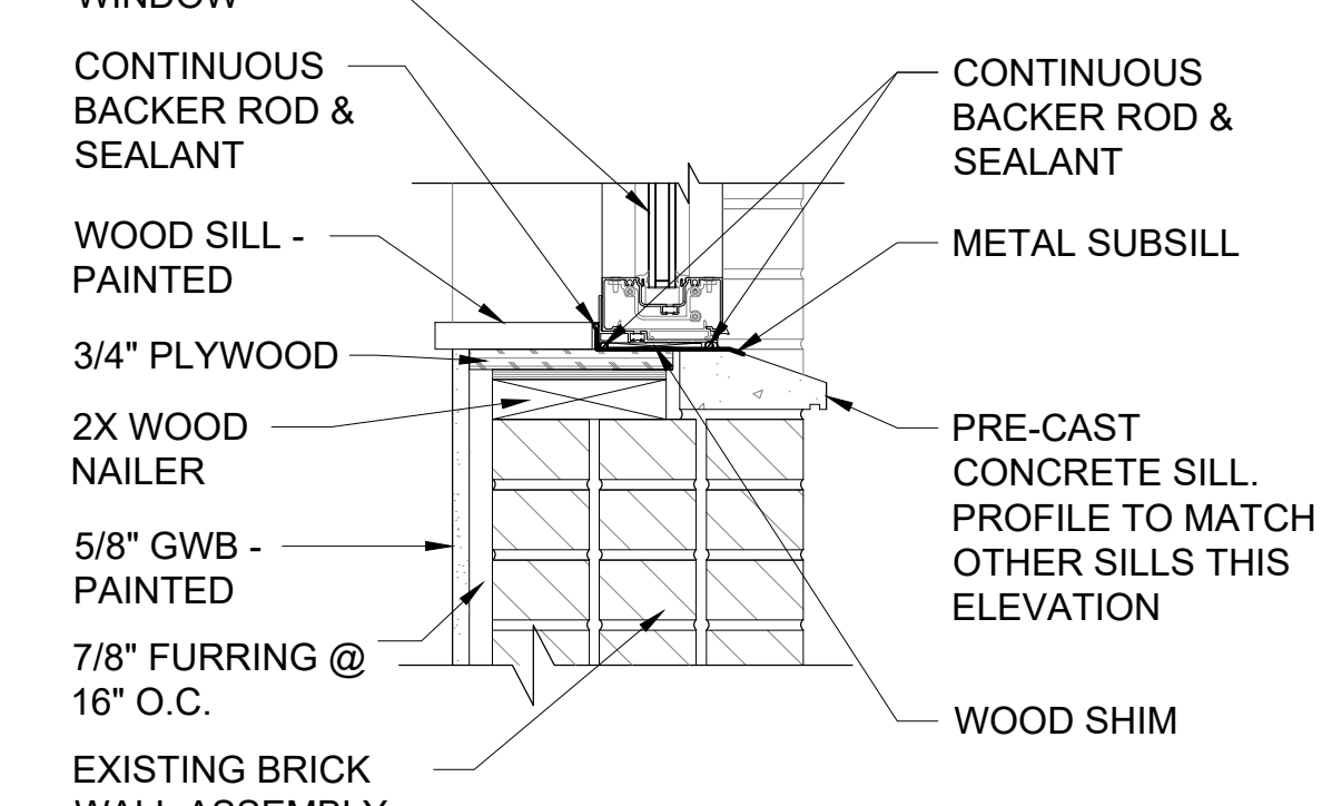
14 WINDOW "J" SILL SCALE: 1-1/2" = 1'-0"
