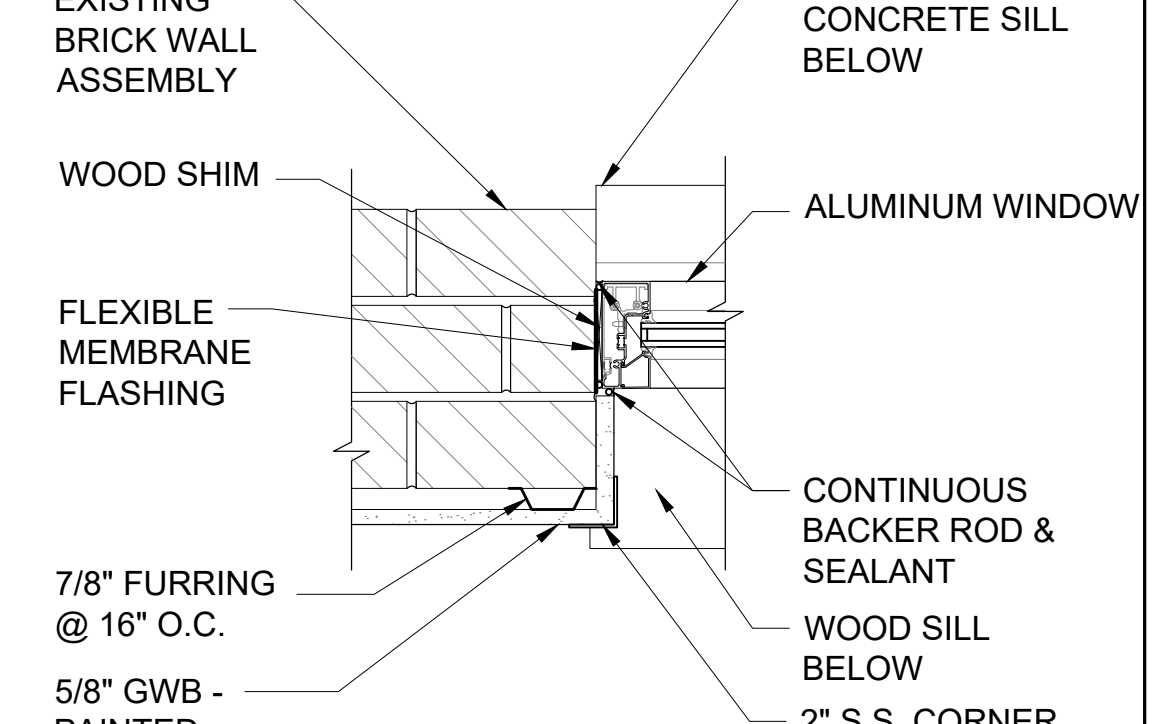
15 WINDOW "J" JAMB SCALE: 1-1/2" = 1'-0"
