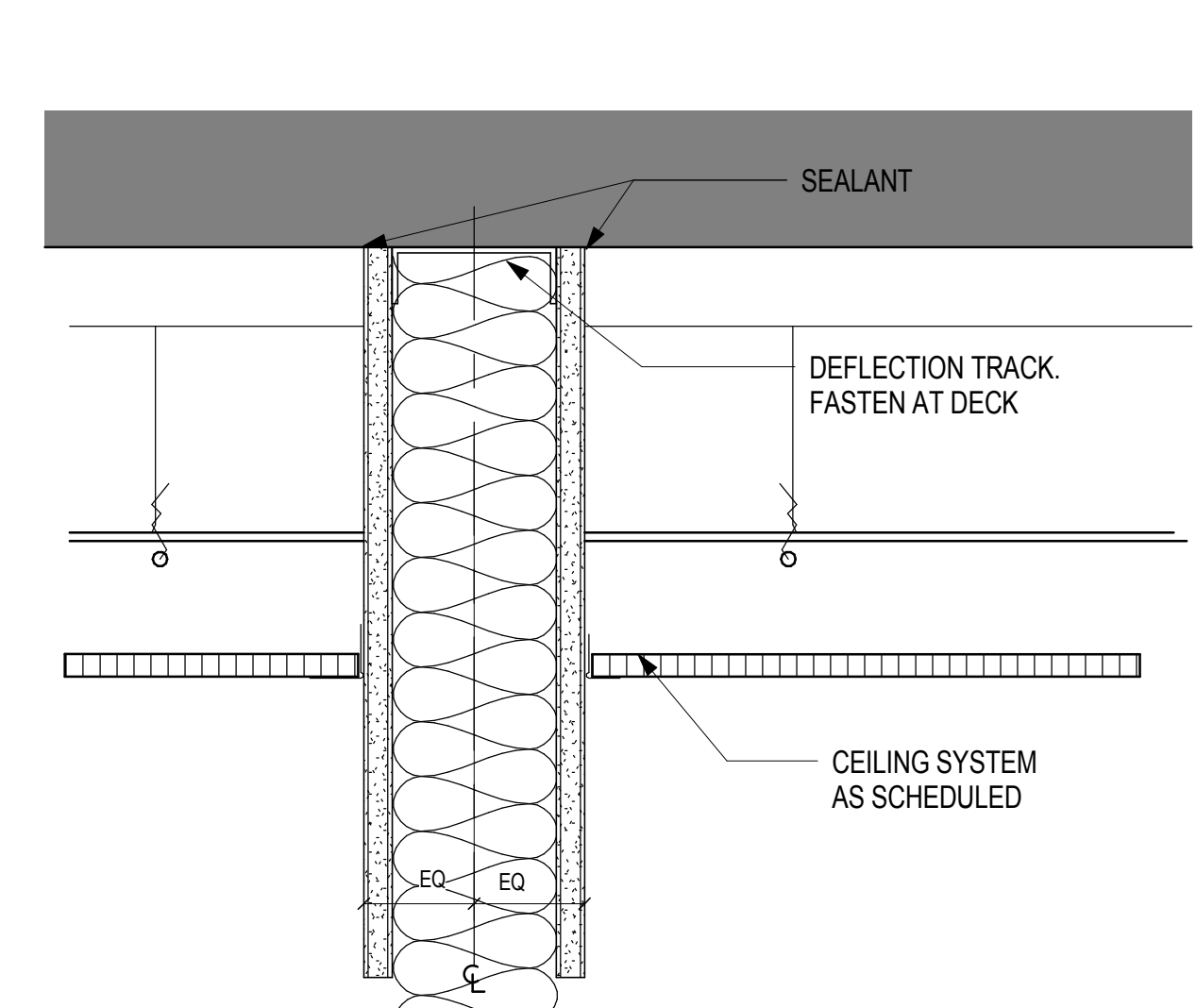
06 HEAD DETAIL - 'HA-02' SCALE: 3" = 1'-0"
