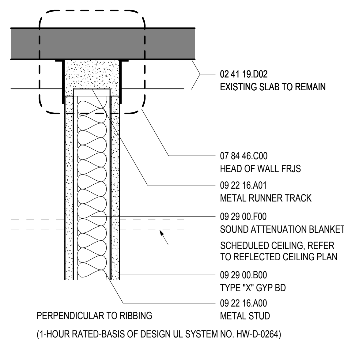
17 HEAD DETAIL 'HA-04' SCALE: 3" = 1'-0"
