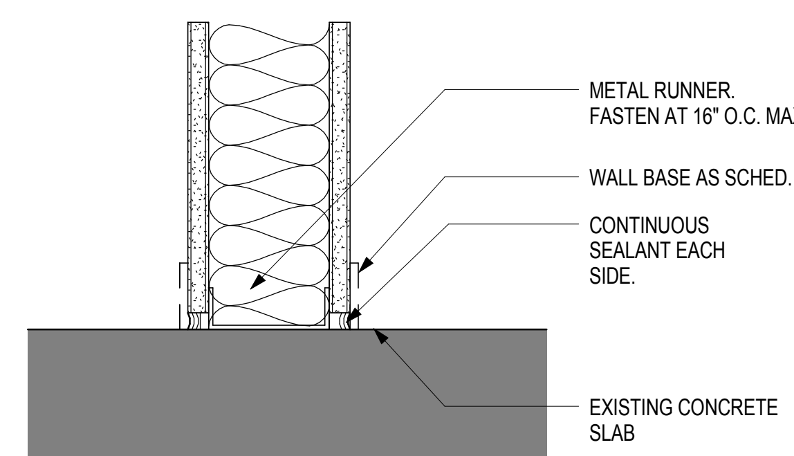
08 BASE DETAIL - 'BA-01' SCALE: 3" = 1'-0"
