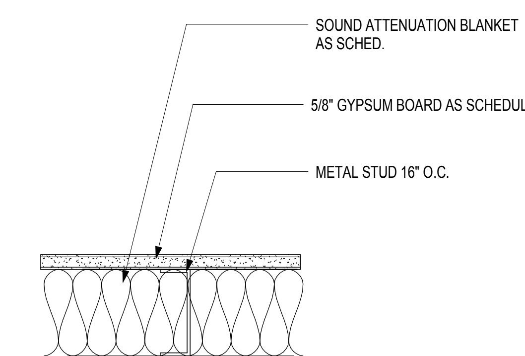
03 PARTITION TYPE - A SCALE: 3" = 1'-0"
