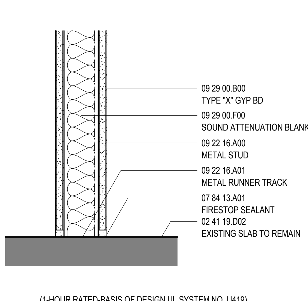
13 BASE DETAIL BA-02 SCALE: 3" = 1'-0"
