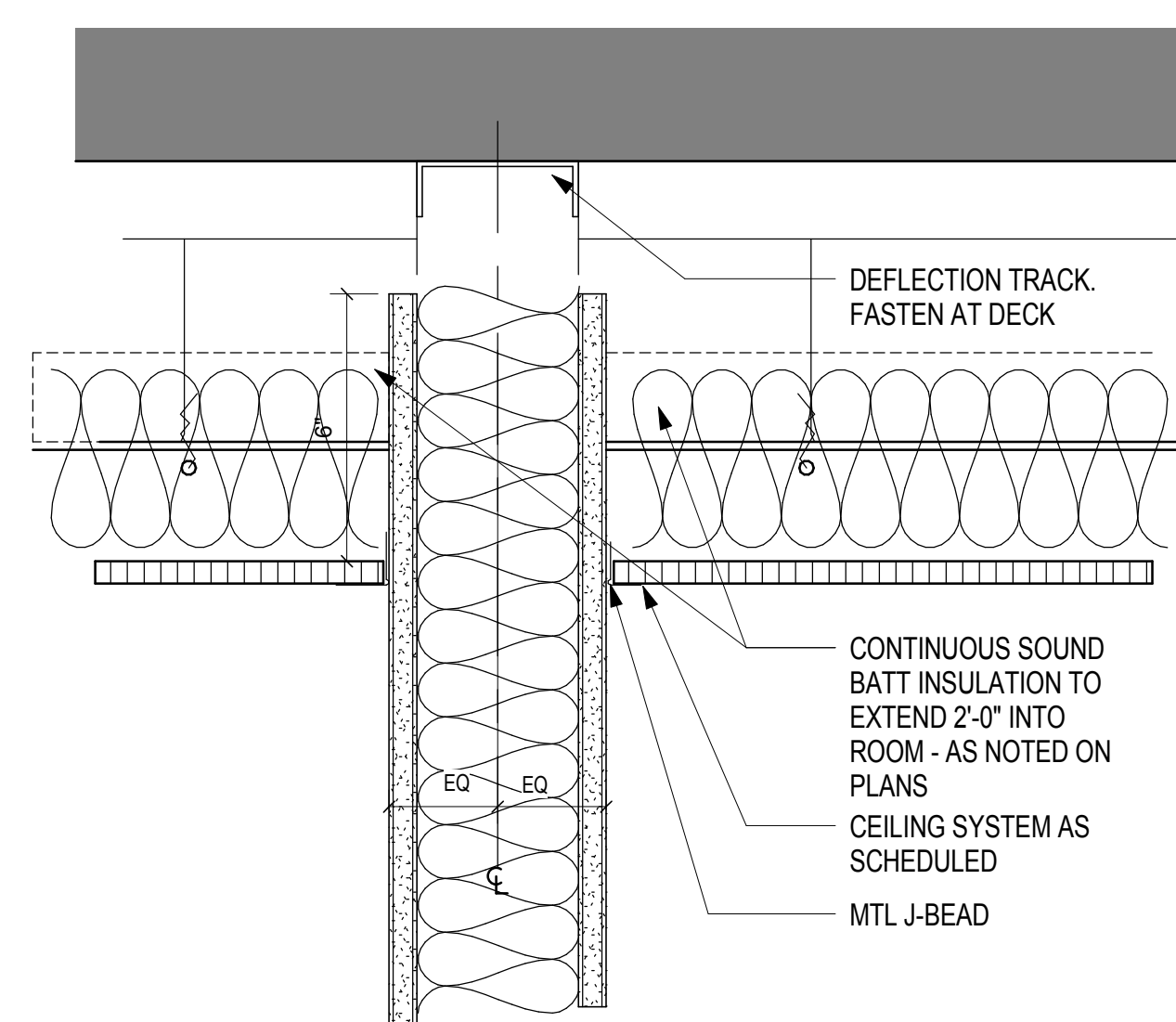
05 HEAD DETAIL - 'HA-01' SCALE: 3" = 1'-0"
