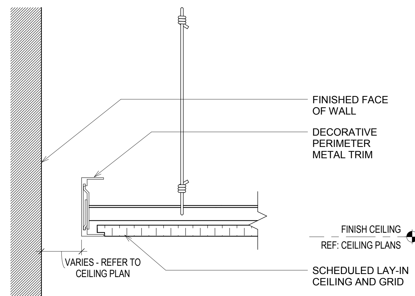
07 CEILING TRIM @ PERIMETER SCALE: 3" = 1'-0"
