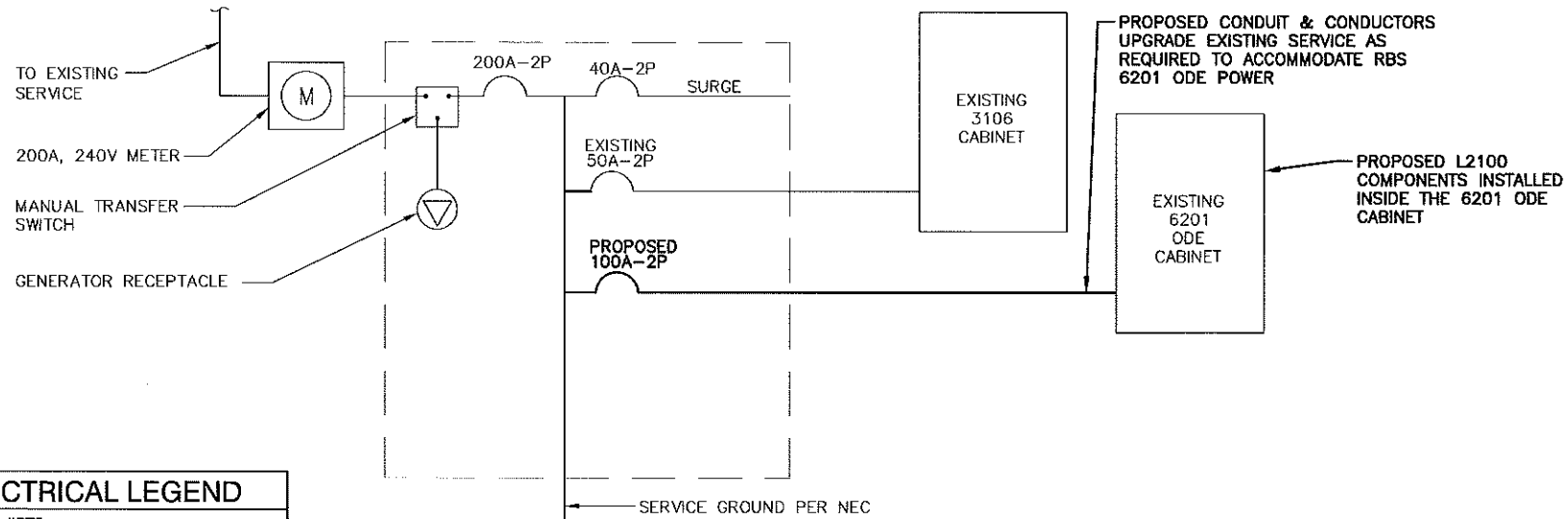
ONE LINE POWER DIAGRAM SCALE: N.T.S.
