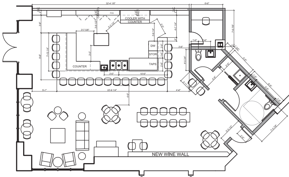
BAR FLOORPLAN 1/4"=1'-0"
