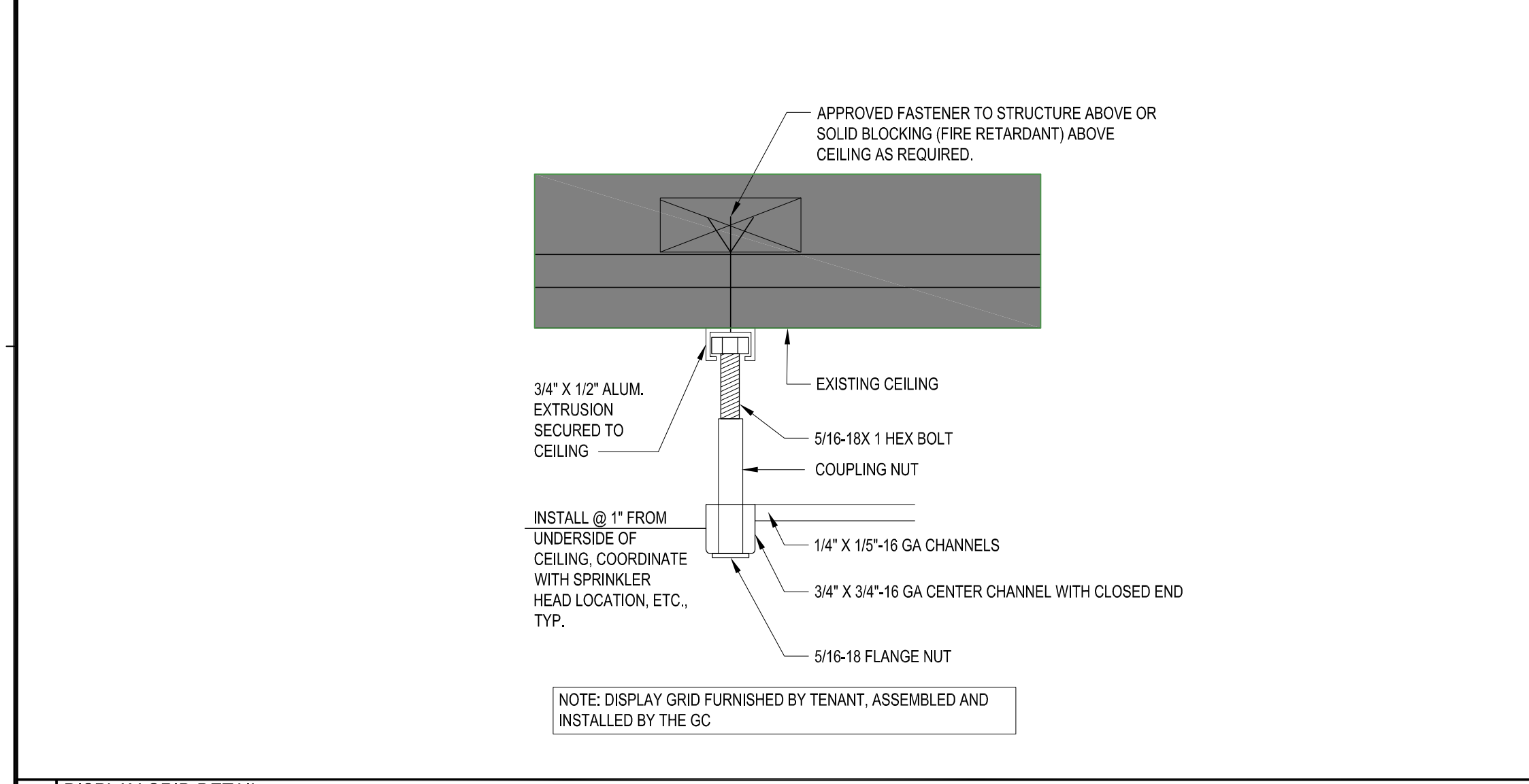
3 DISPLAY GRID DETAIL SCALE: 6" = 1'-0"
