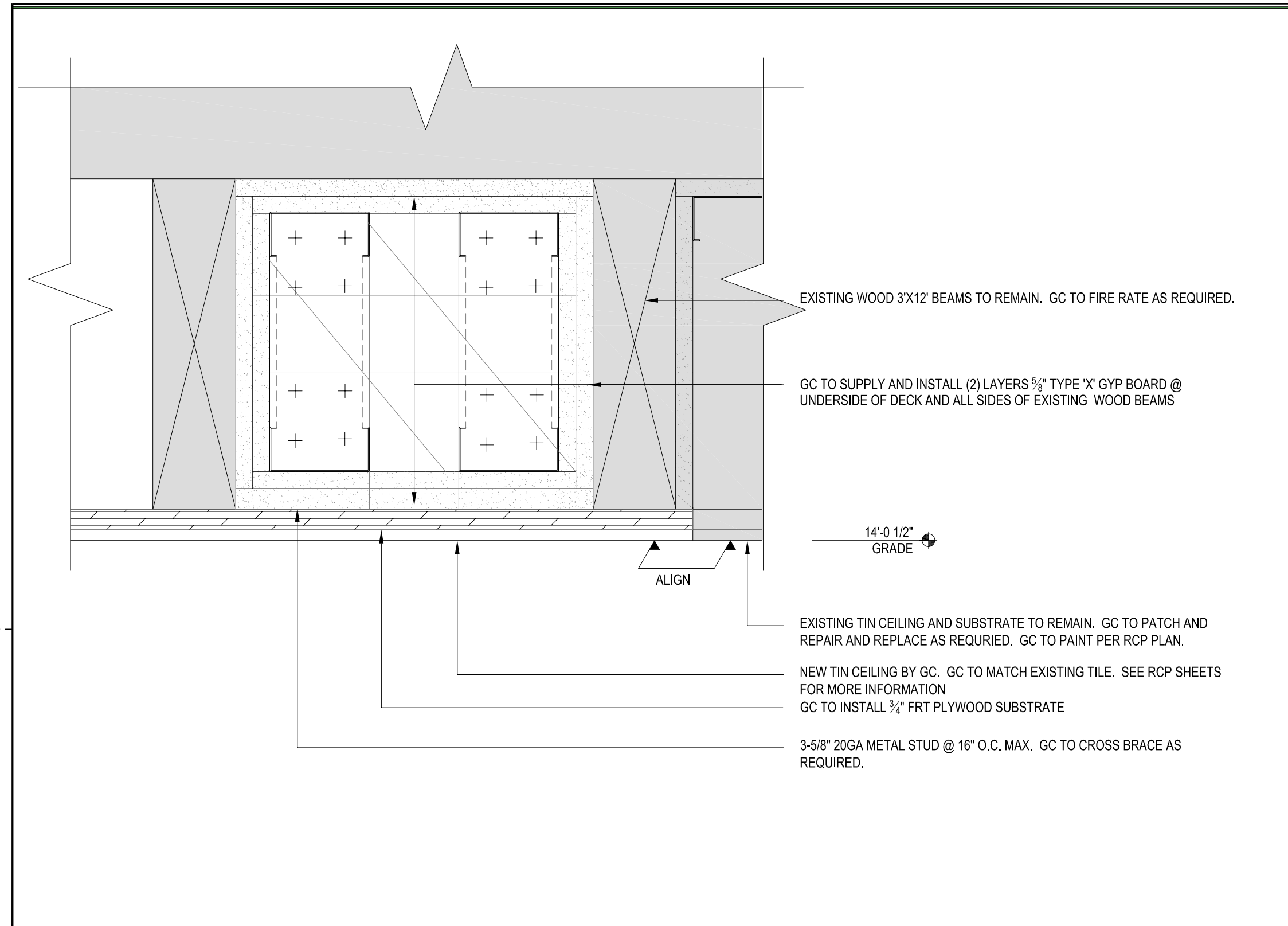
1 CEILING DETAIL SCALE: 3" = 1'-0"
