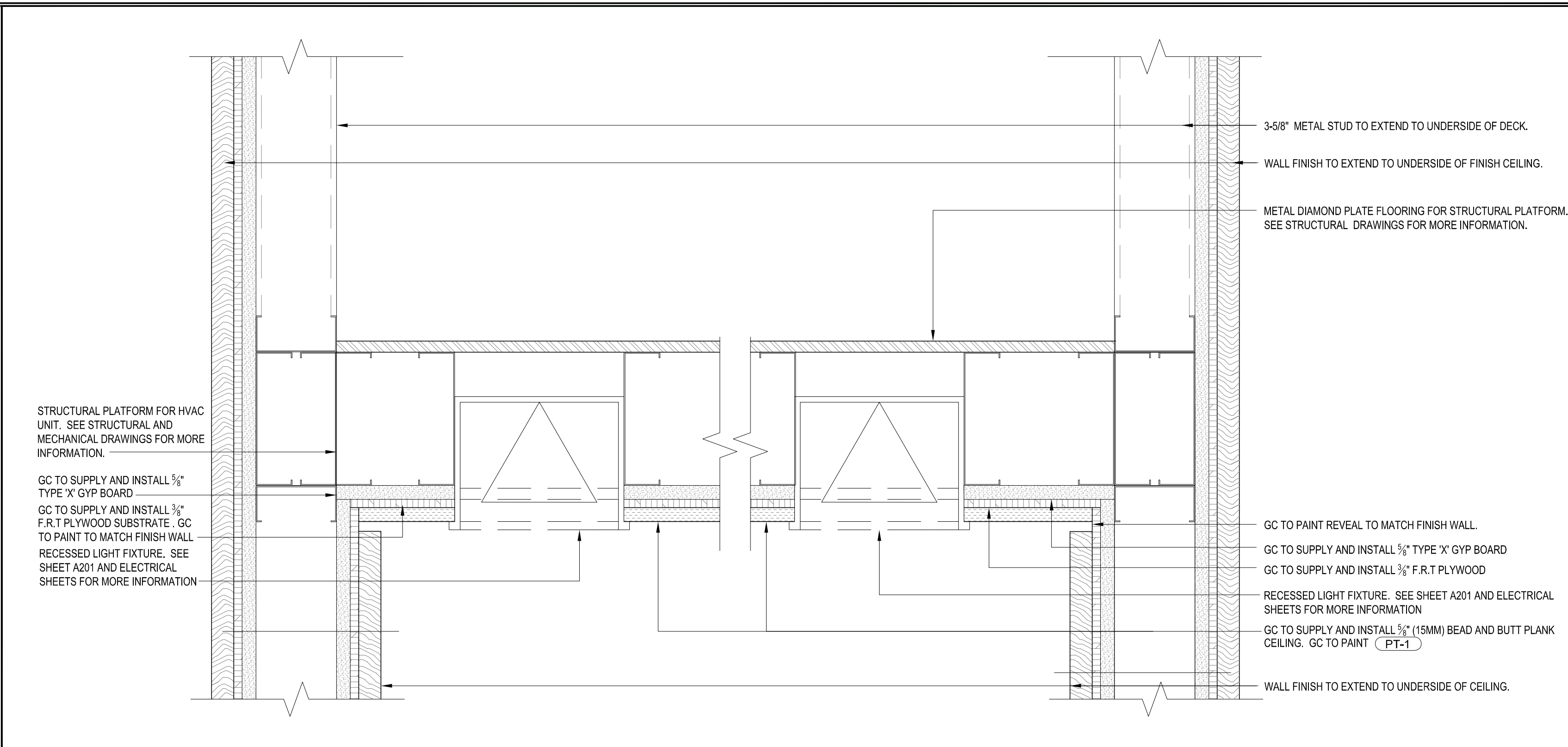
2 CEILING DETAIL SCALE: 3" = 1'-0"
