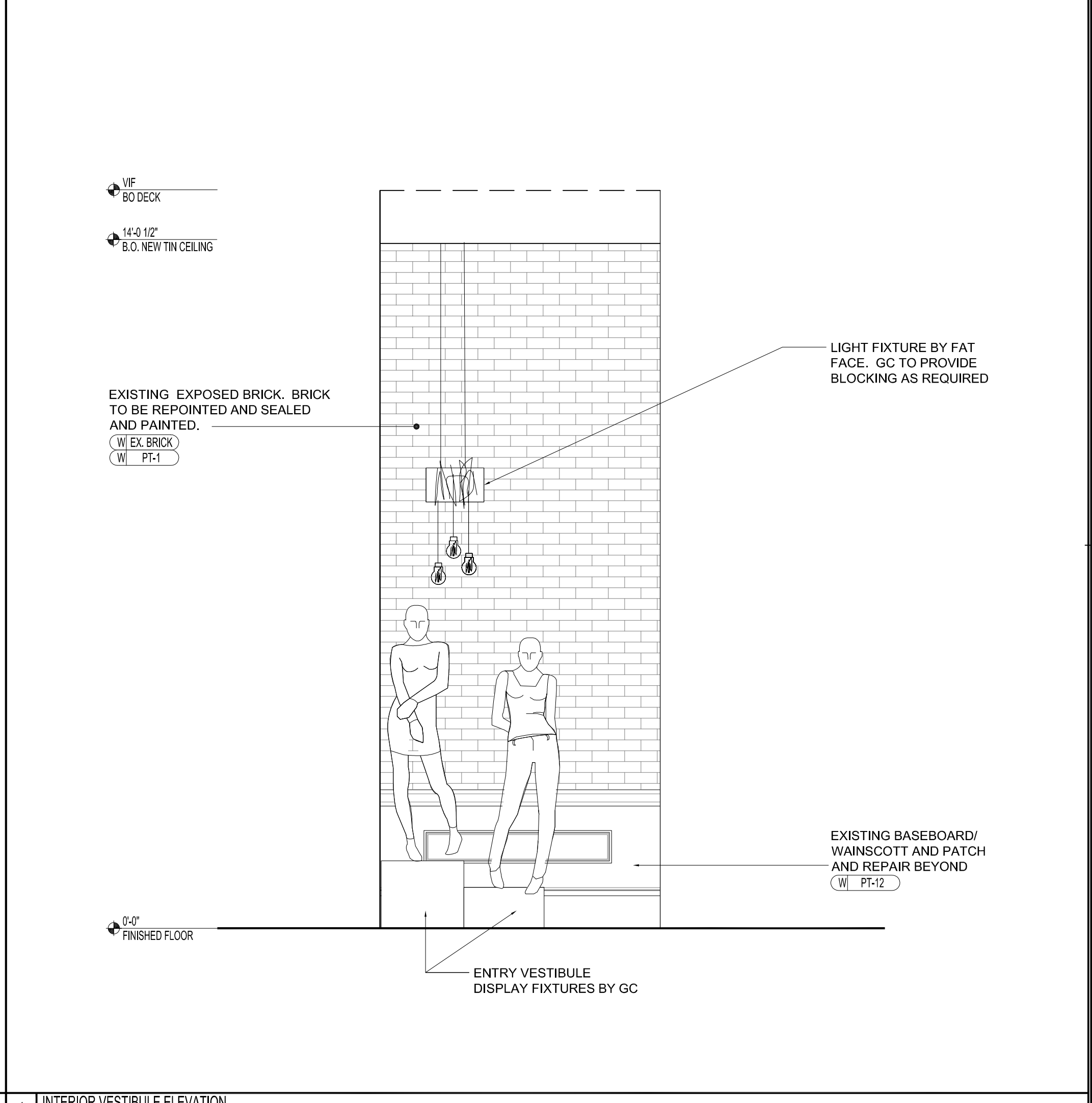
4 INTERIOR VESTIBULE ELEVATION SCALE: 1/2" = 1'-0"
