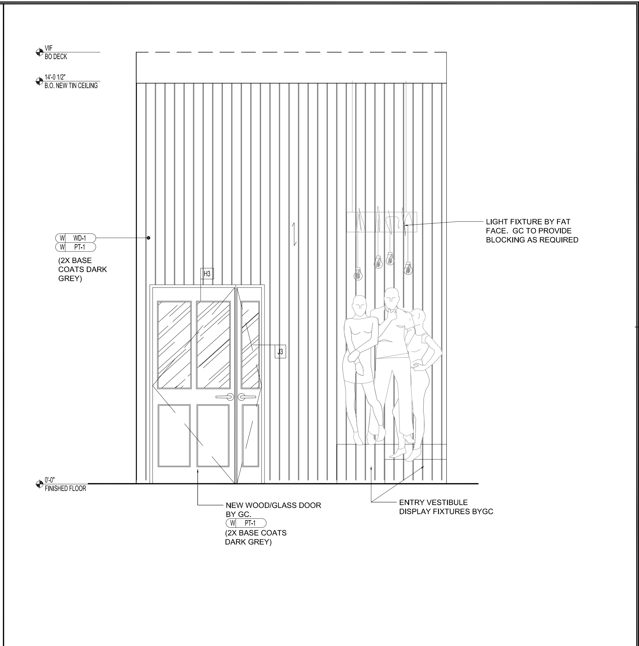
3 INTERIOR VESTIBULE ELEVATION SCALE: 1/2" = 1'-0"
