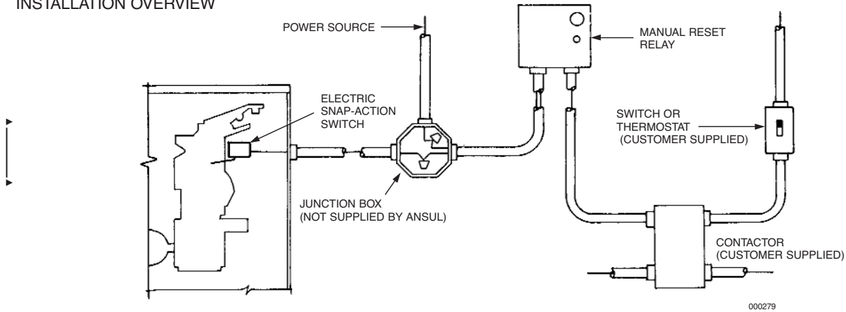
WIRING SCHEMATIC
