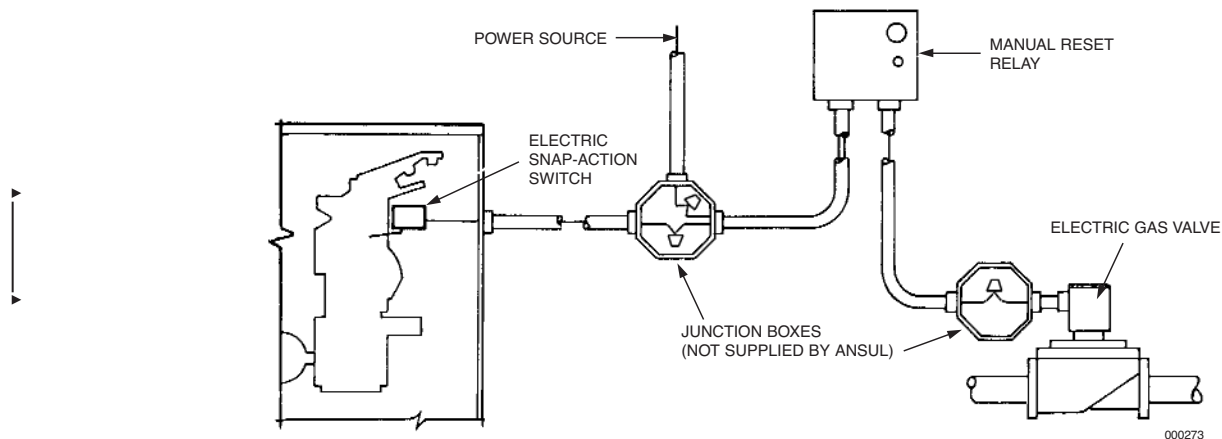
WIRING SCHEMATIC
