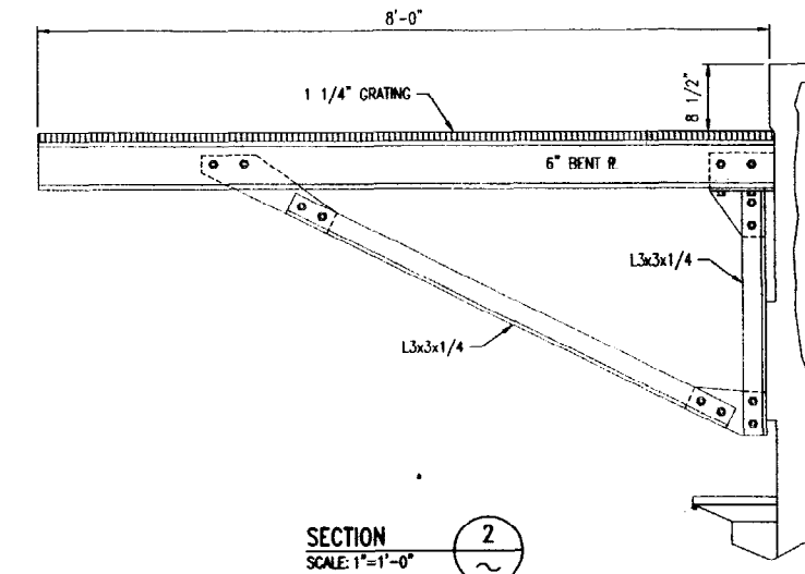
SECTION 1 SCALE: 1"=1'-0"
