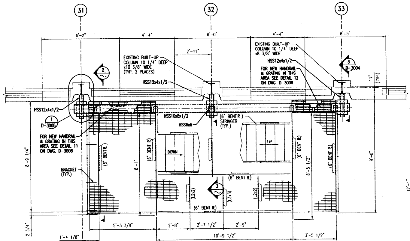
LEVEL 2 SCALE: 1/2"=1'-0"
