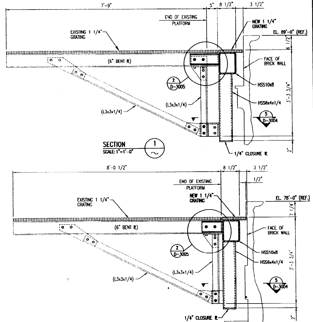
SECTION 2 SCALE: 1"=1'-0"
