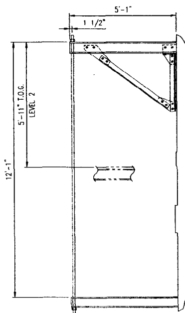
SECTION 3 SCALE: 1/2"=1'-0"
