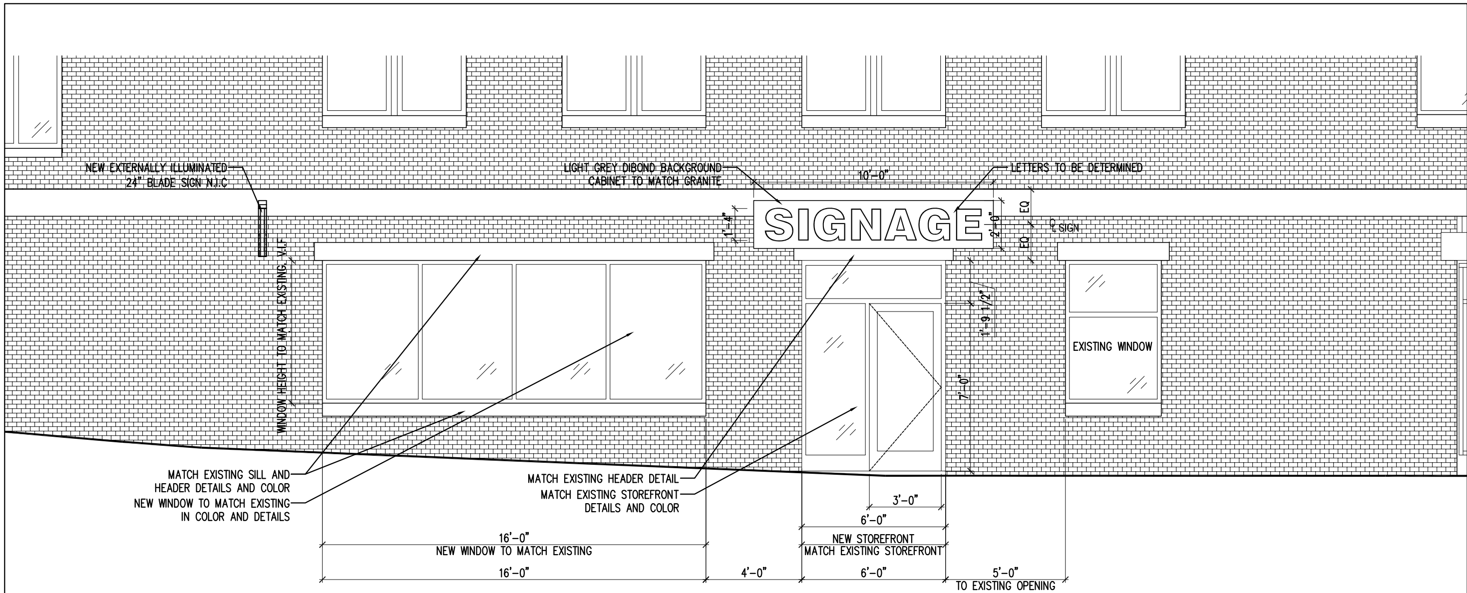
1 | ENLARGED STOREFRONT SCALE: 1/4"=1'-0"
