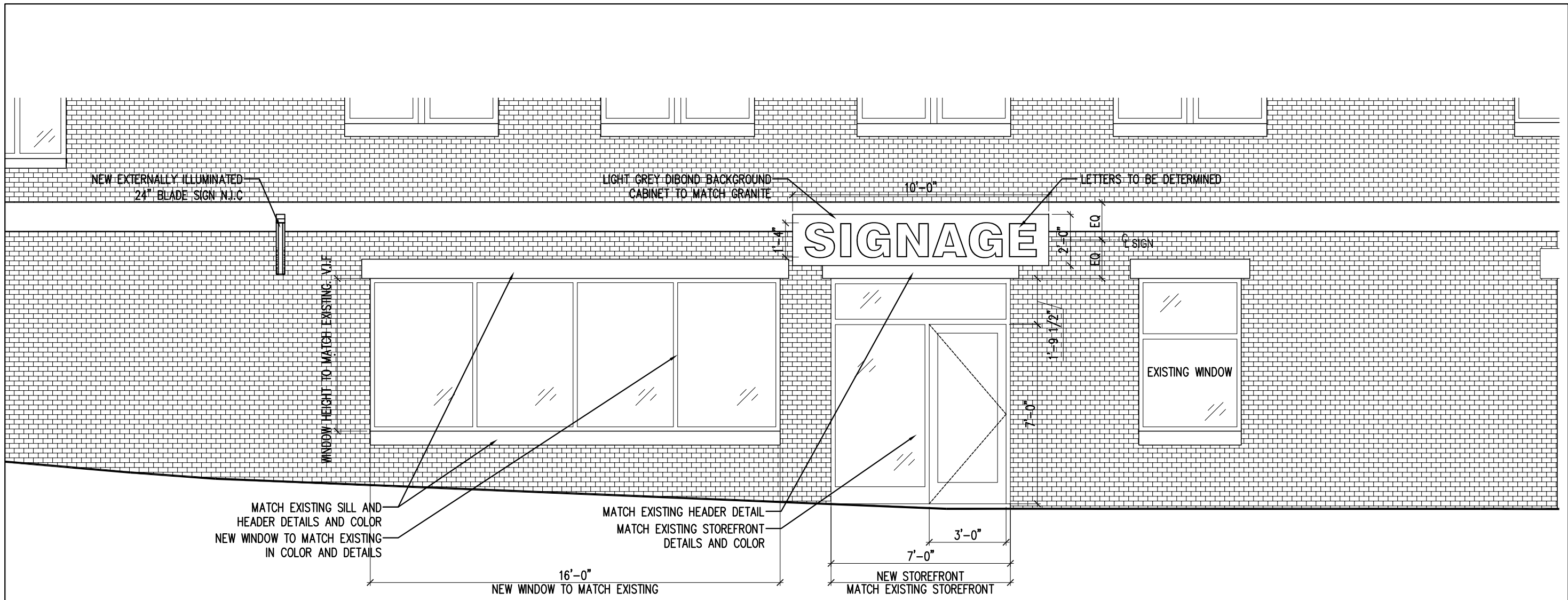
1 | ENLARGED STOREFRONT SCALE: 1/4"=1'-0"
