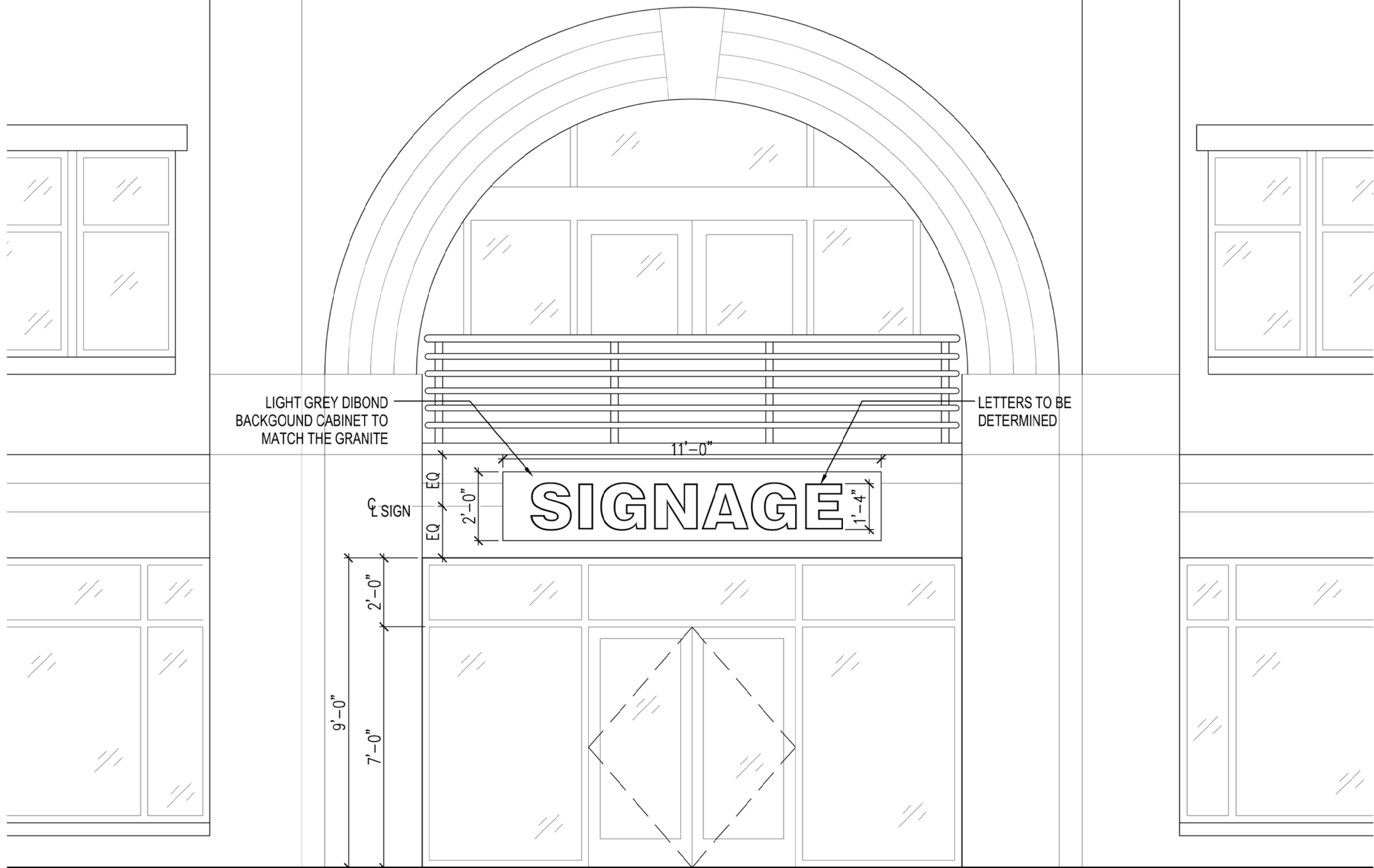
1 ENLARGED CENTER STOREFRONT ELEVATION SCALE: 3/8" = 1'-0"
