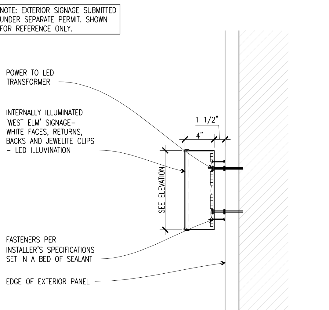
A3 WALL-MOUNTED SIGNAGE 1 1/2"=1'-0" SIGNAGE FOIO
