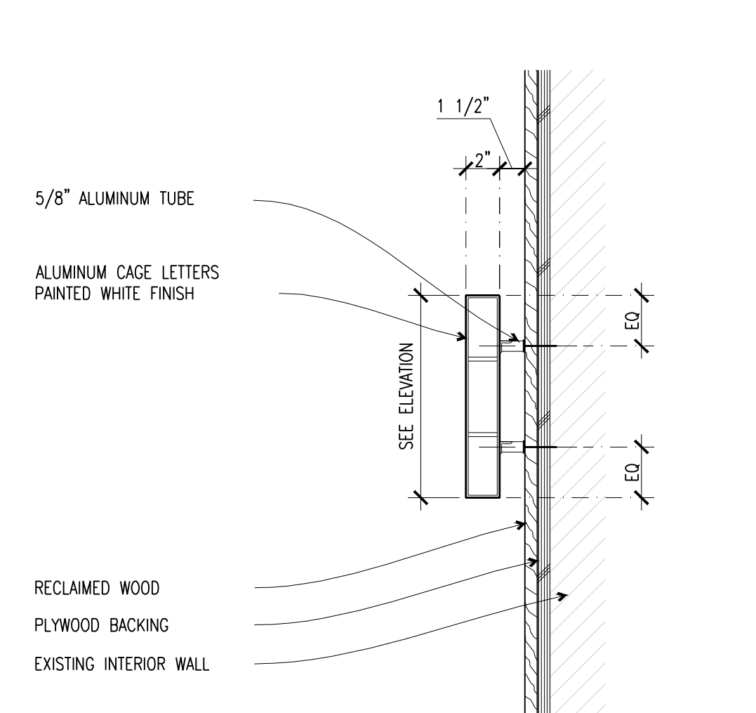
A5 WALL-MOUNTED CAGE SIGNAGE 1 1/2"=1'-0" SIGNAGE FOIO
