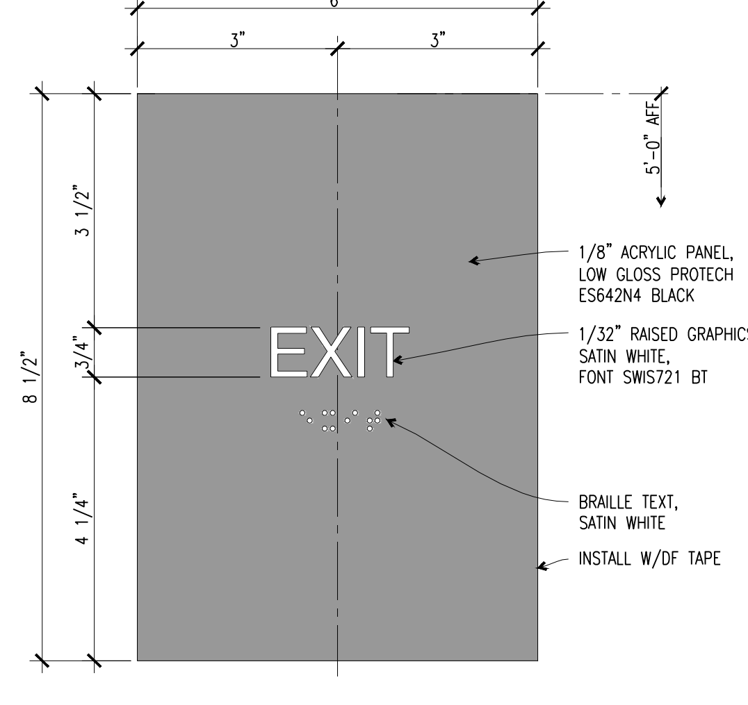
A7 TACTILE EXIT SIGNAGE 6"=1'-0" SIGNAGE FOIO
