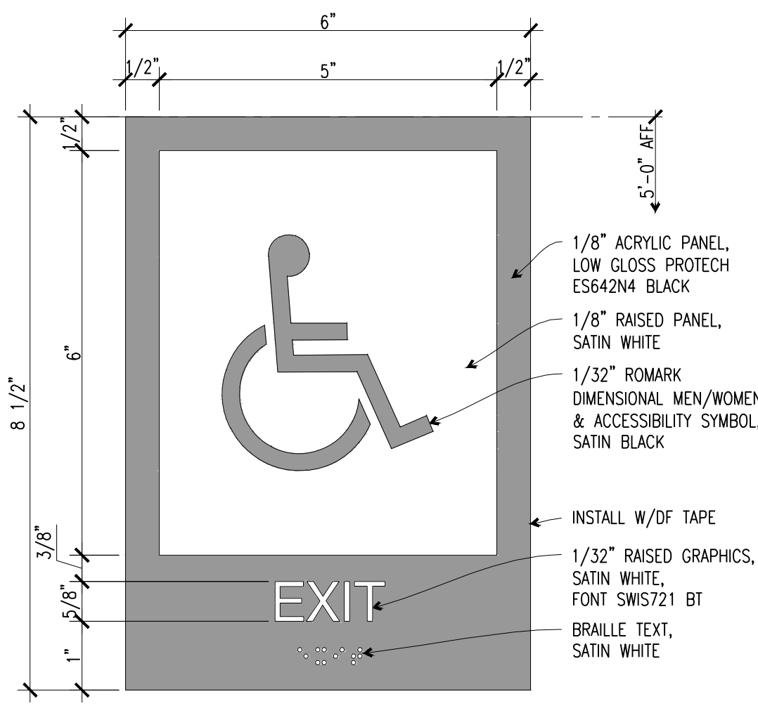
C3 ACCESSIBLE EXIT SIGNAGE 6"=1'-0" SIGNAGE FOIO
