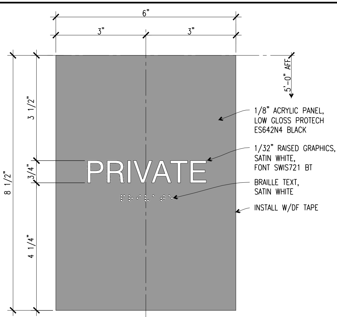
E3 PRIVATE SIGNAGE 6"=1'-0" SIGNAGE FOIO
