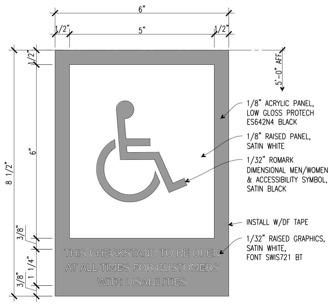
C1 ACCESSIBLE CASHWRAP SIGN 6"=1'-0" SIGNAGE FOIO
