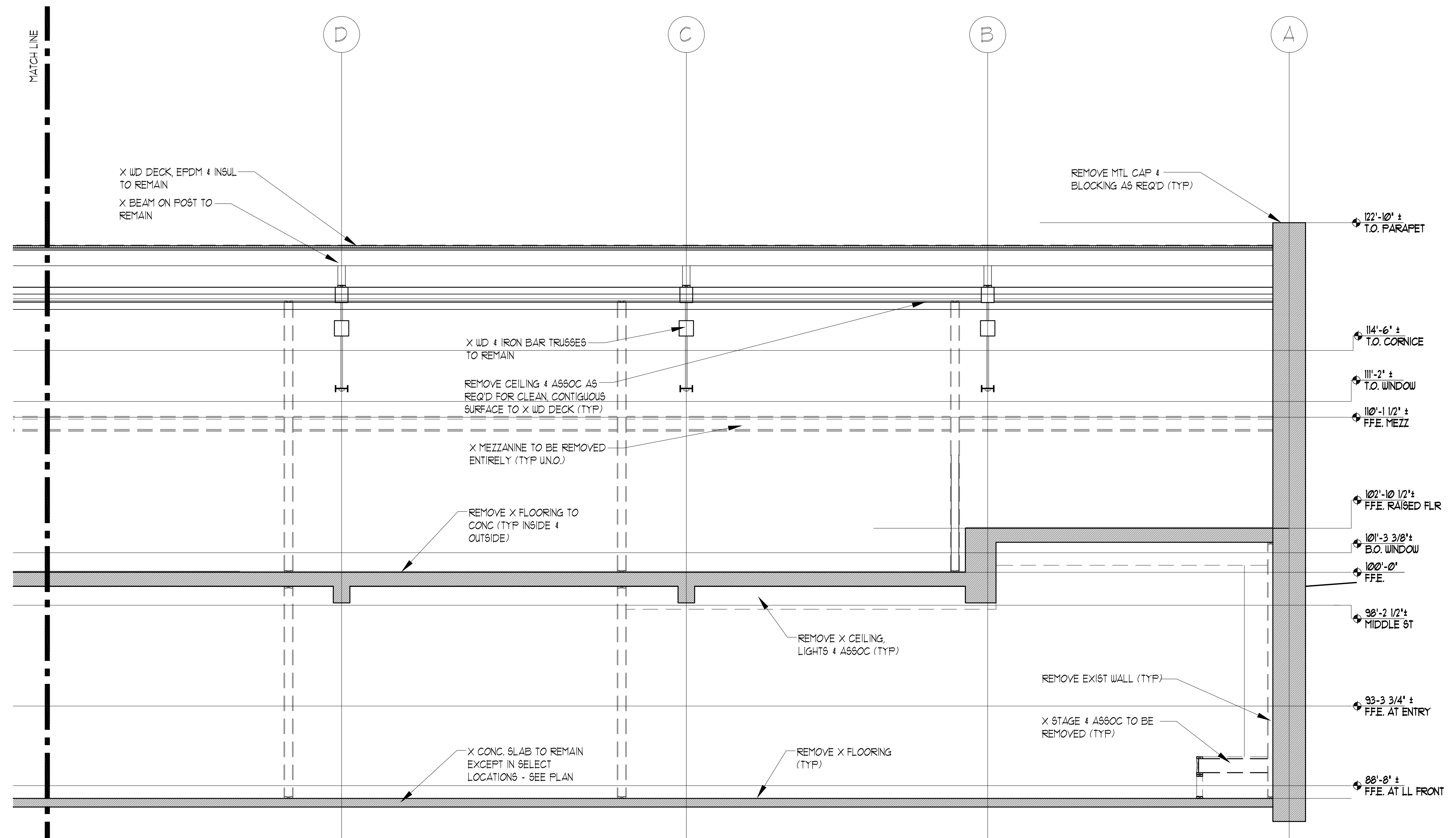
DEMO BUILDING SECTION D11D3.4 SCALE: 1/8" = 1'-0"
