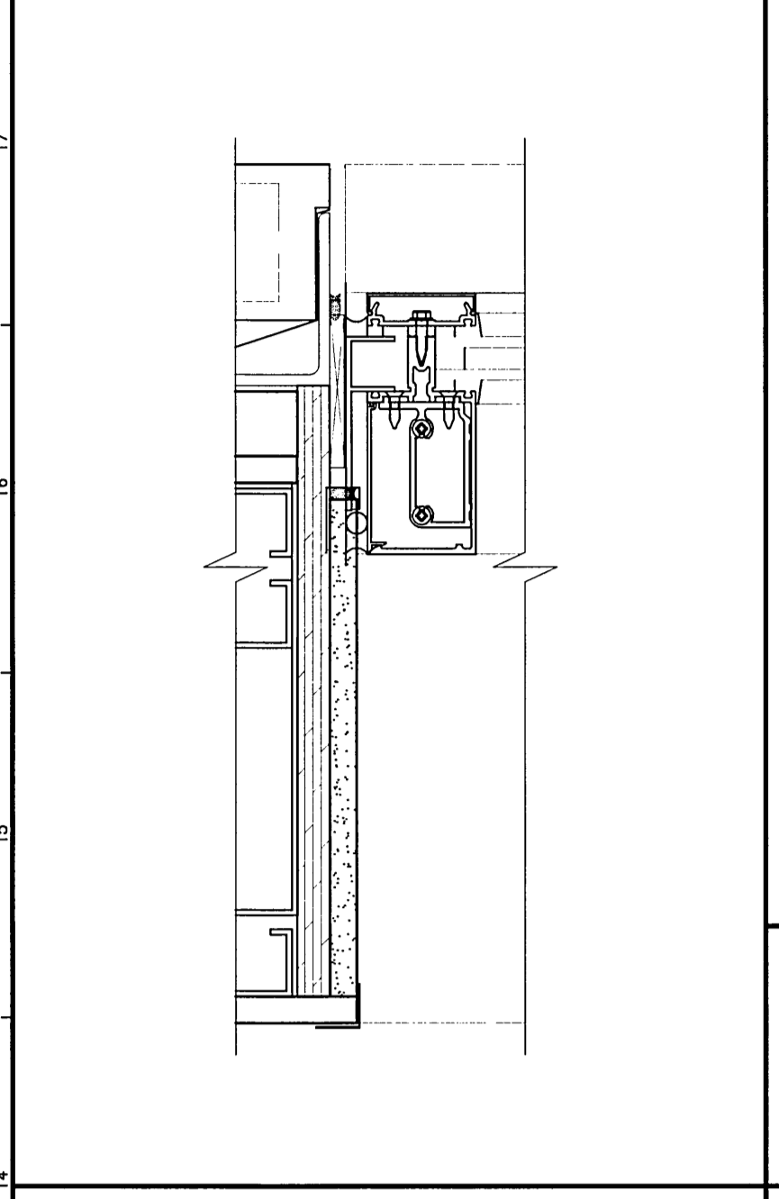
P14 JAMB DETAIL 3"=1'-0"
