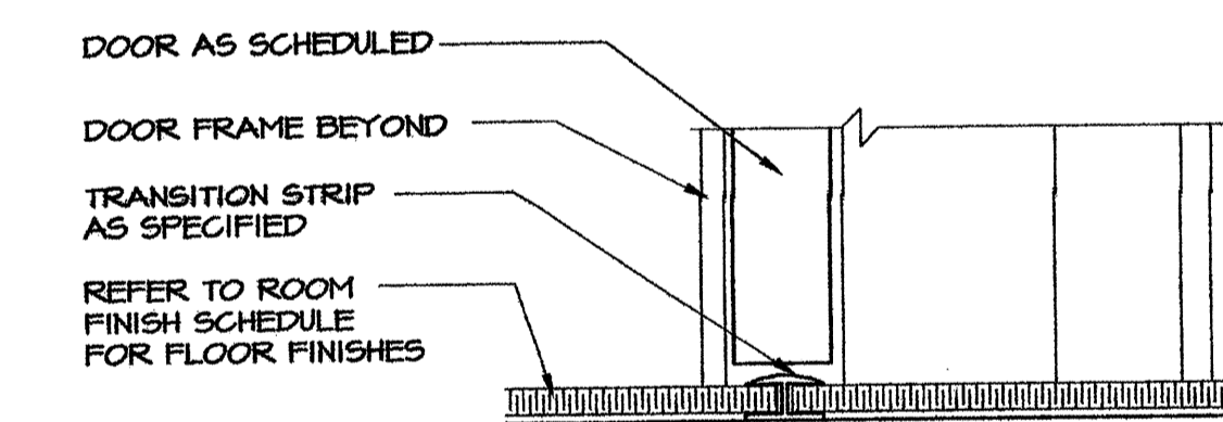
S1 SILL DETAIL SCALE: 3" = 1'-0"
