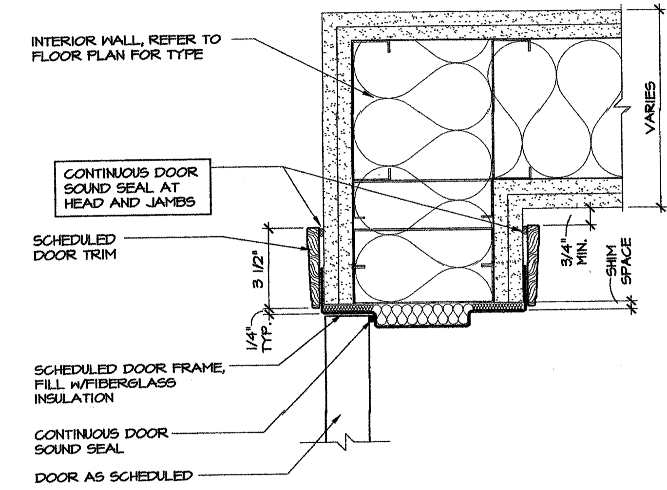
J1 JAMB DETAIL SCALE: 3" = 1'-0"
