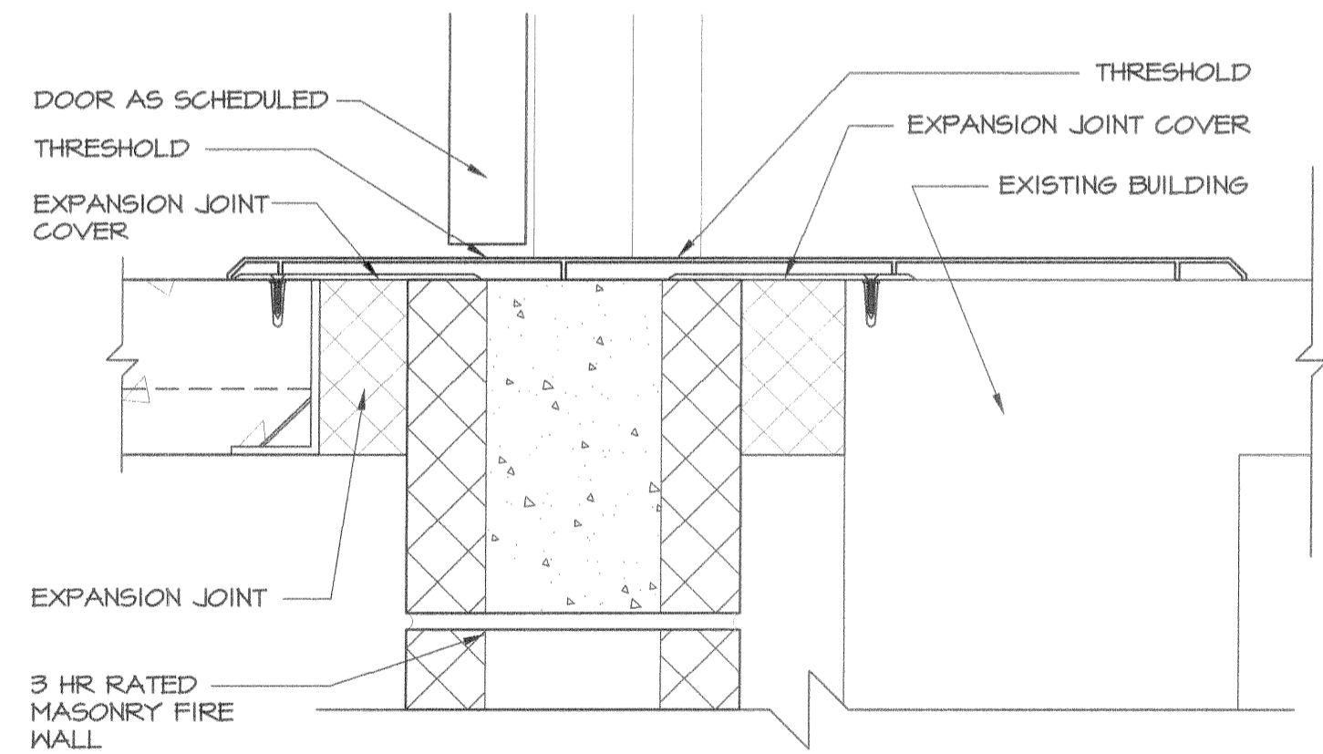
S2 SILL DETAIL SCALE: 3" = 1'-0"
