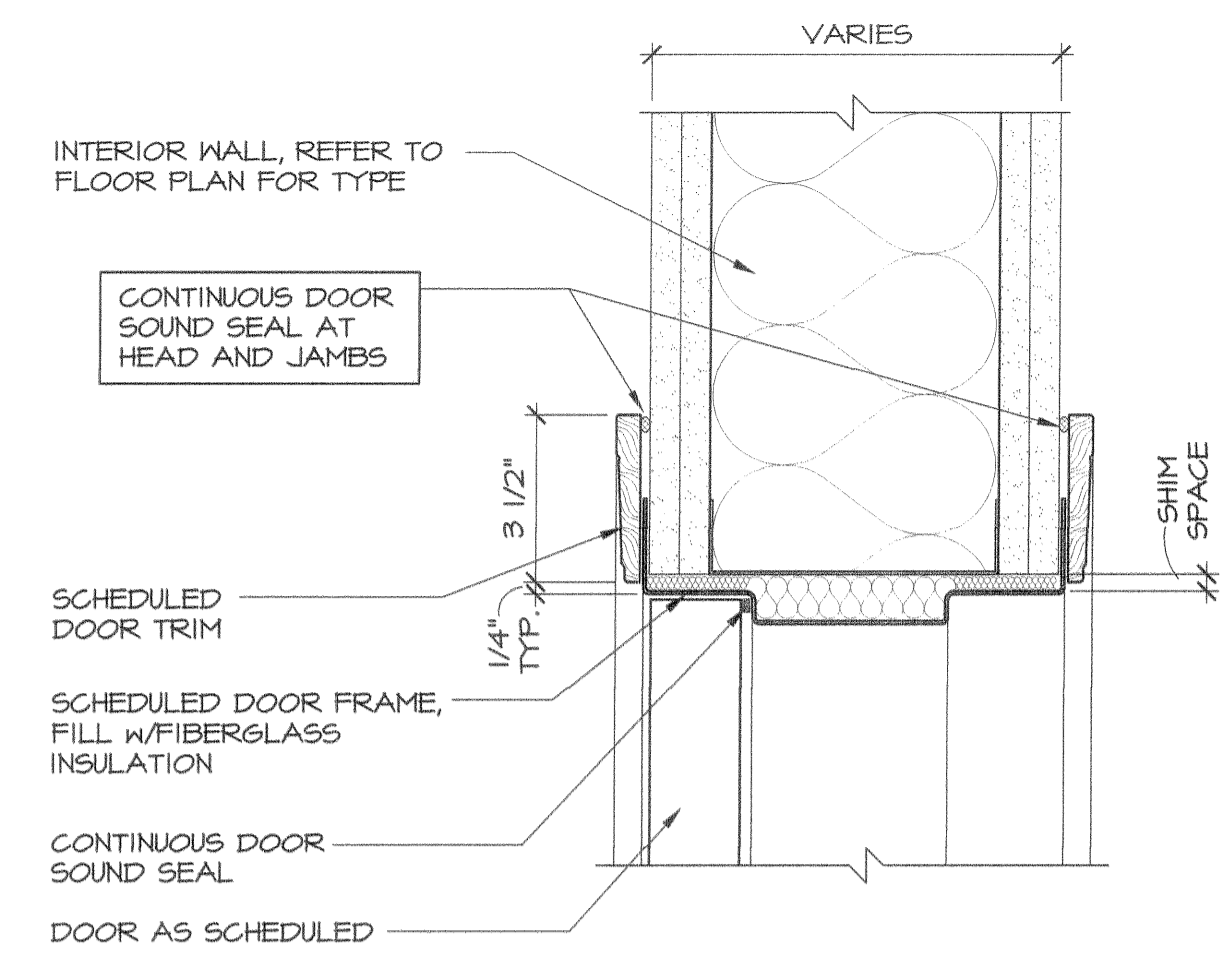
H1 HEAD DETAIL SCALE: 3" = 1'-0"
