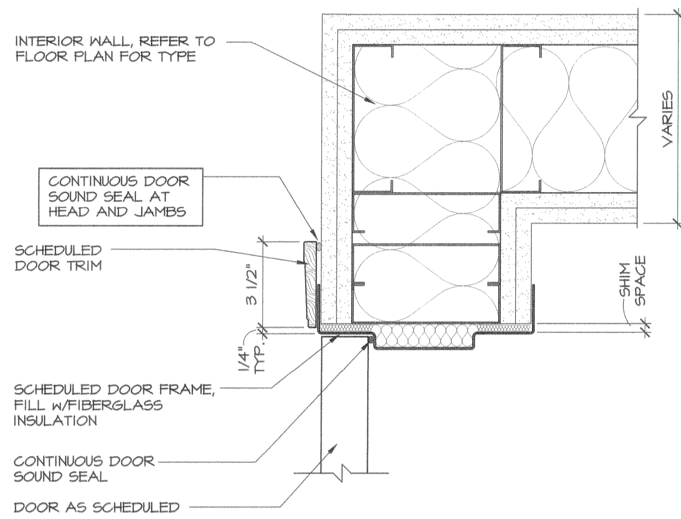
J4 JAMB DETAIL SCALE: 3" = 1'-0"
