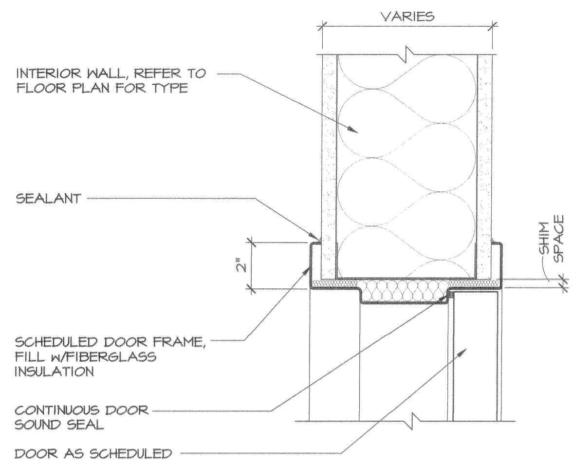
H2 HEAD DETAIL SCALE: 3" = 1'-0"
