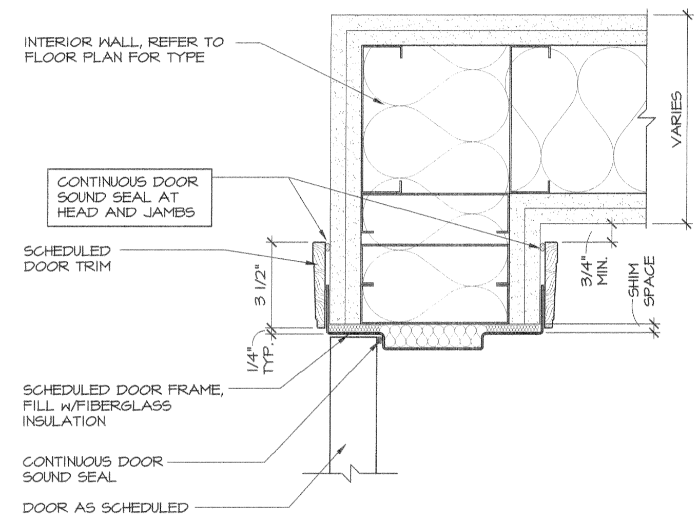
J1 JAMB DETAIL SCALE: 3" = 1'-0"
