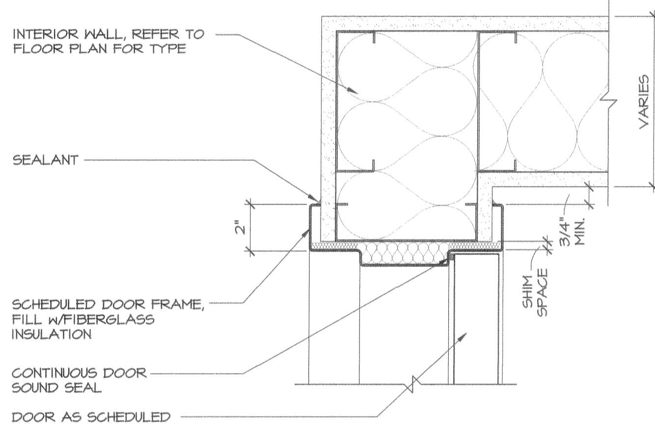
J2 JAMB DETAIL SCALE: 3" = 1'-0"
