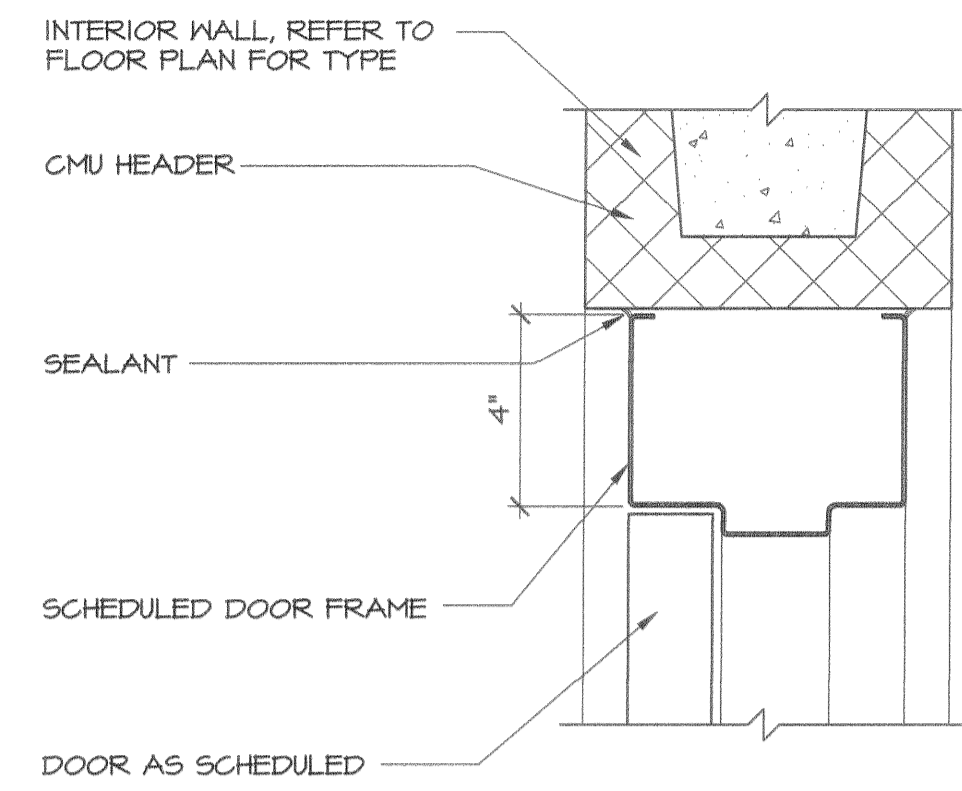
H3 HEAD DETAIL SCALE: 3" = 1'-0"
