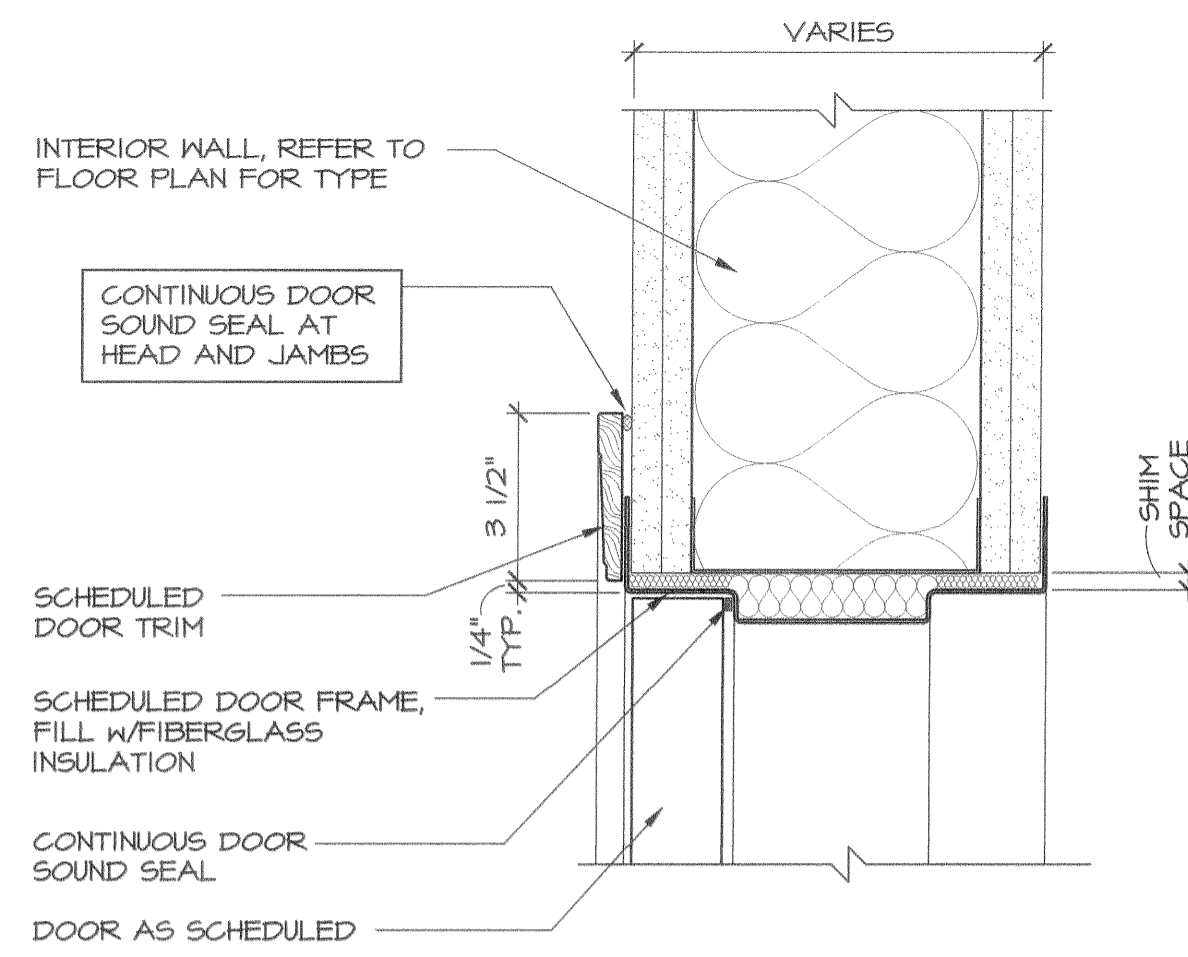
H4 HEAD DETAIL SCALE: 3" = 1'-0"
