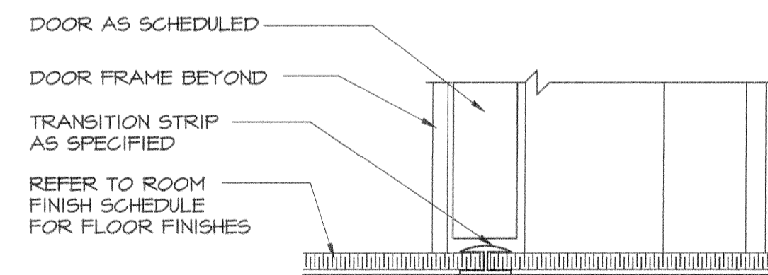
S1 SILL DETAIL SCALE: 3" = 1'-0"
