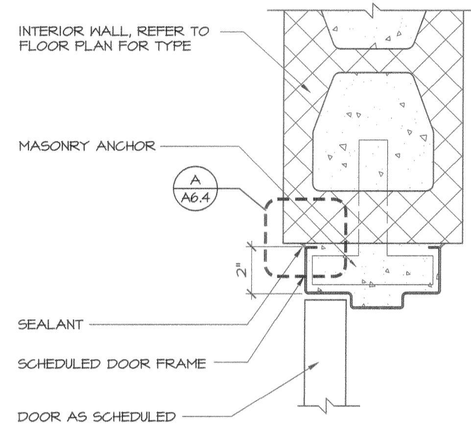
J3 JAMB DETAIL SCALE: 3" = 1'-0"
