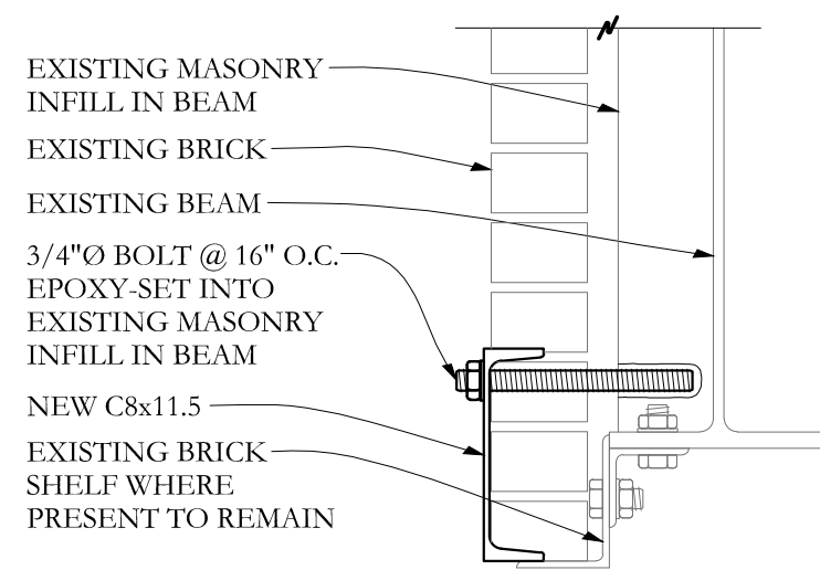
SECTION C S3.1 1 1/2"=1'-0
