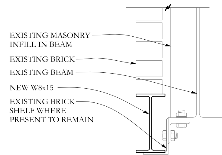
SECTION D S3.1 1 1/2"=1'-0
