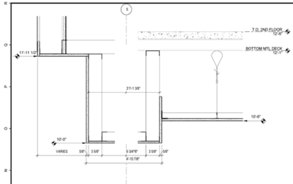
M1 CEILING DETAIL - 1
