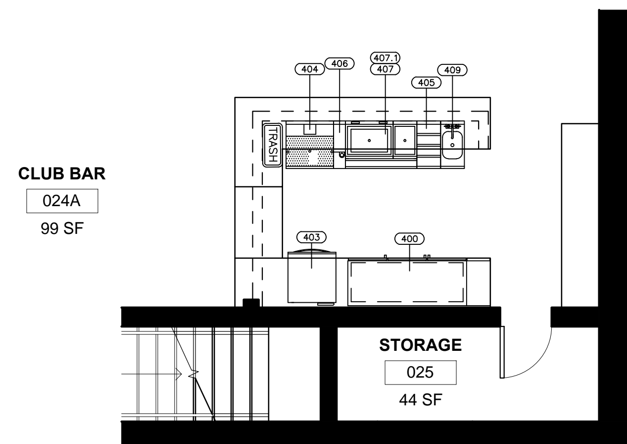
Bar 400 Scale: 1/4"=1'-0"
