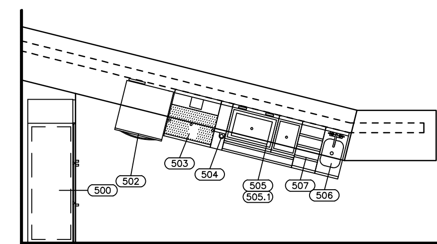
Bar 500 Scale: 1/4"=1'-0"
