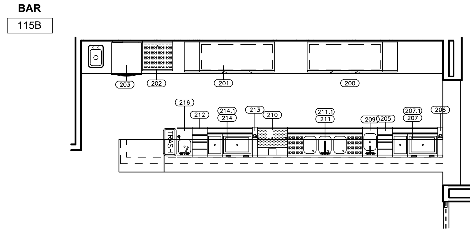
Bar 200 Scale: 1/4"=1'-0"
