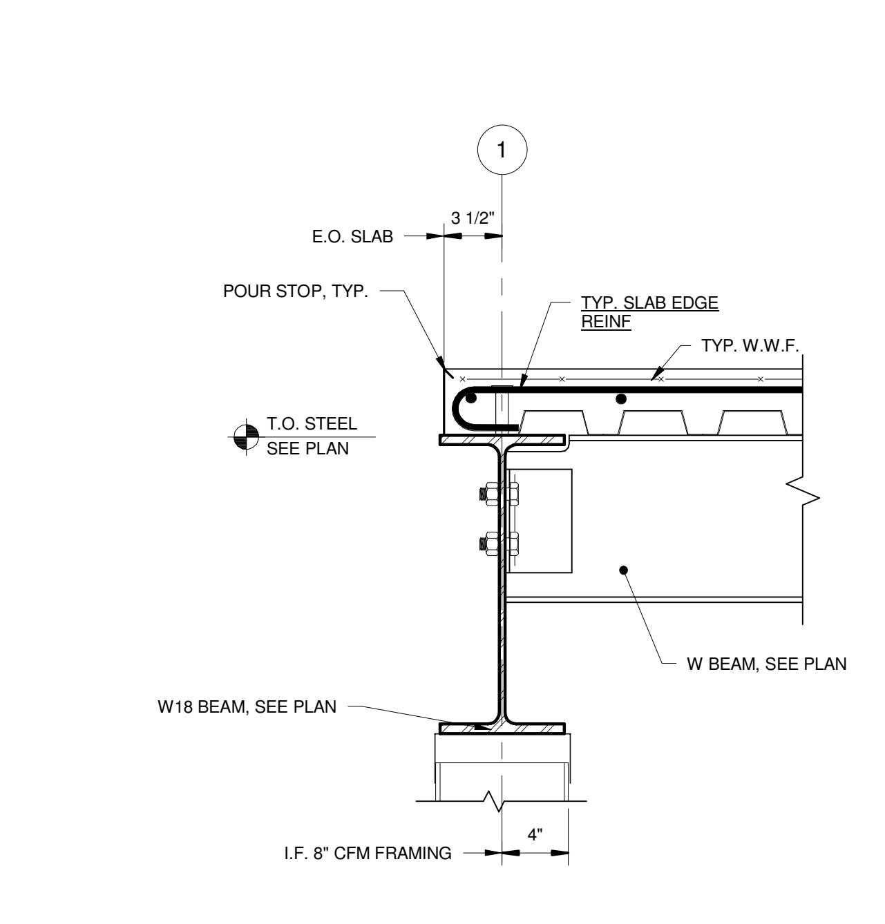
E1 SECTION 1 1/2" = 1'-0"
