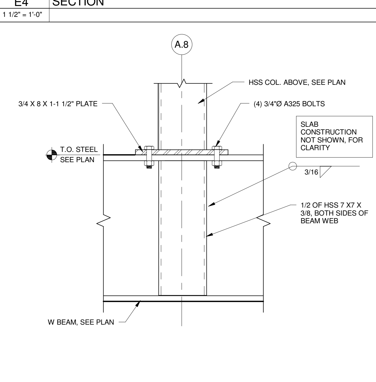
A4 SECTION 1 1/2" = 1'-0"
