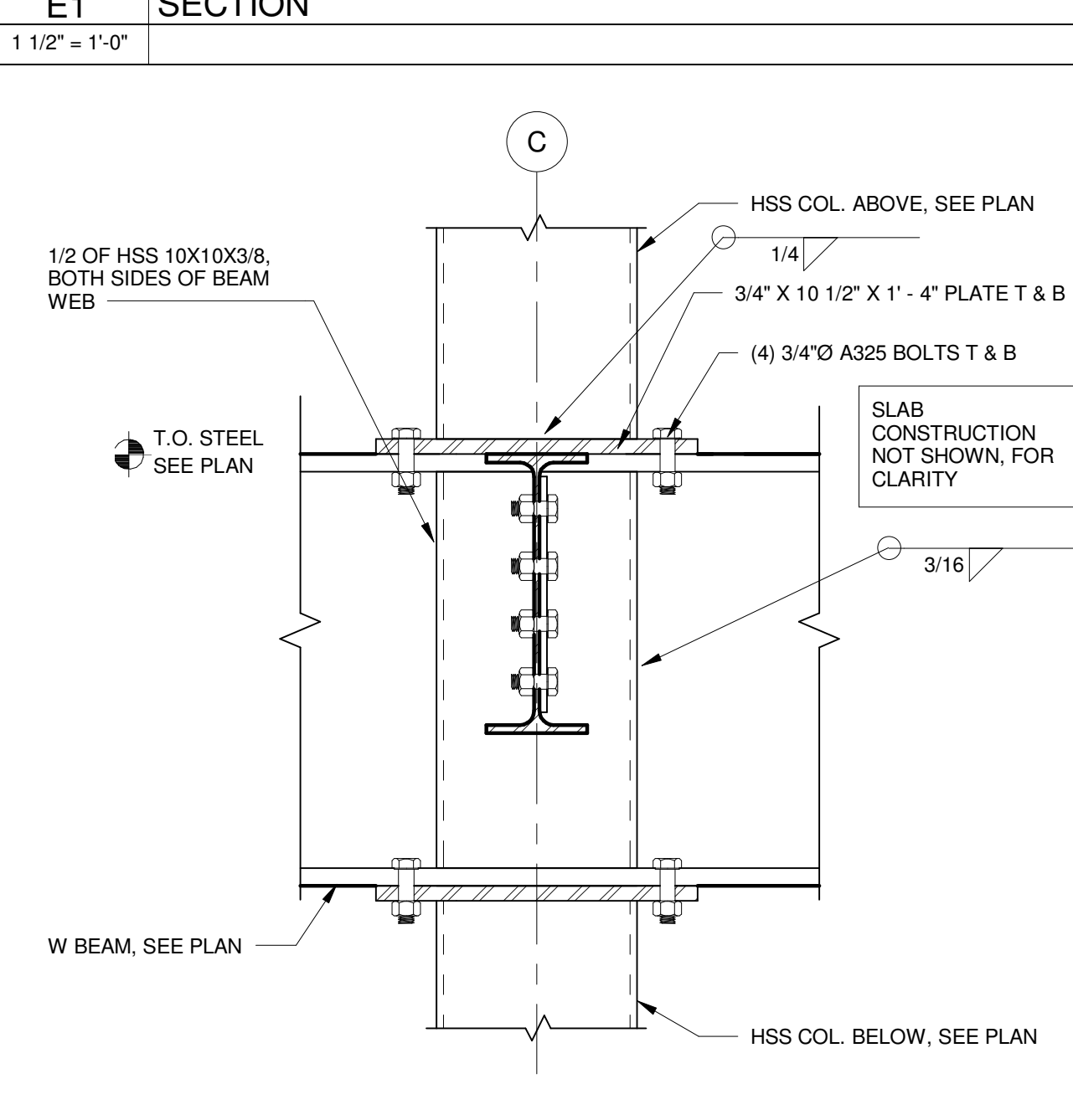
A1 SECTION 1 1/2" = 1'-0"
