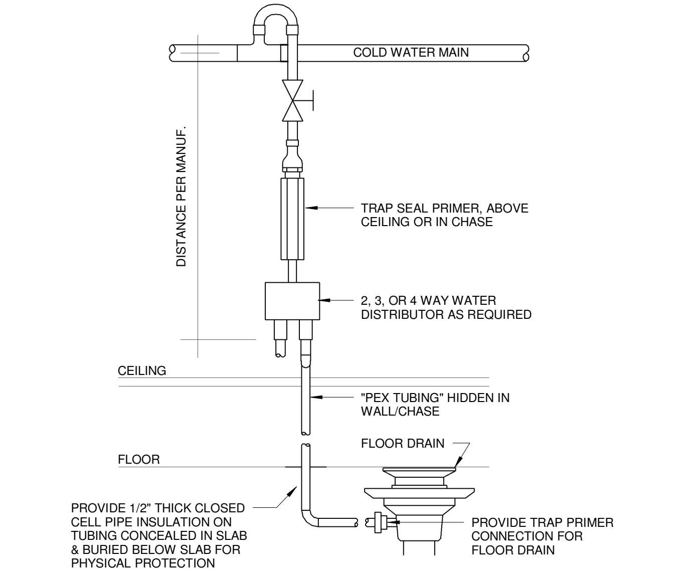
A12 TRAP PRIMER DETAIL NTS
