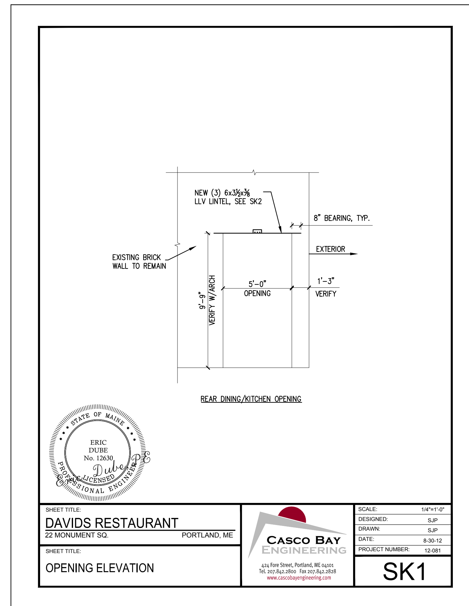
1 Davids SK1 SCALE: 1" = 1'-0"
