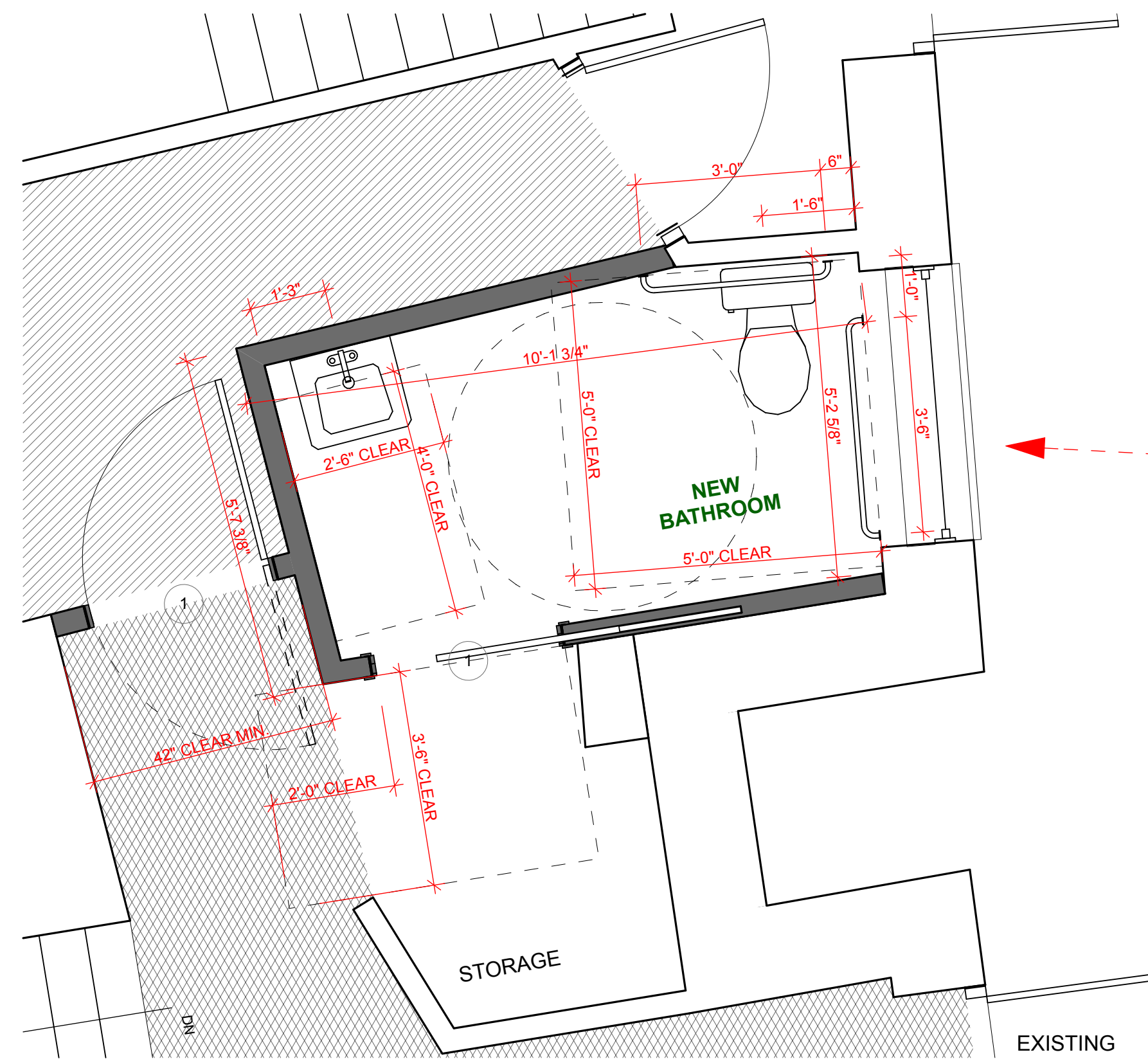
2 NEW BATHROOM SCALE: 1/2" = 1'-0"
