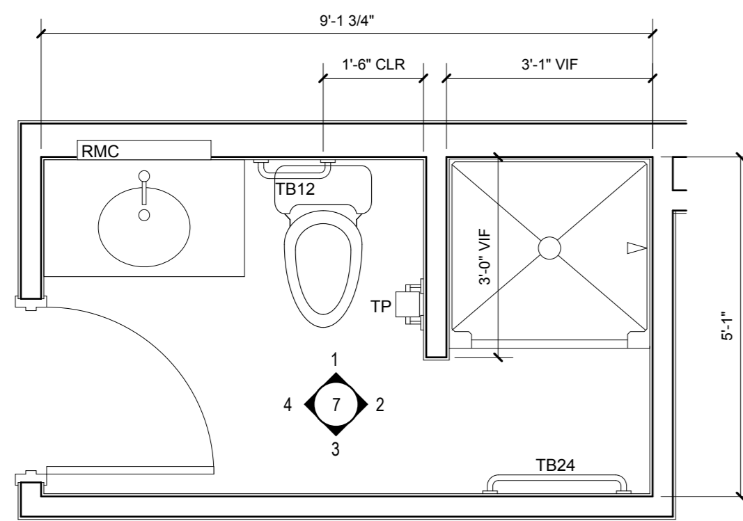
7 BATHROOM TYPE "G" SCALE: 1/2" = 1'-0"
