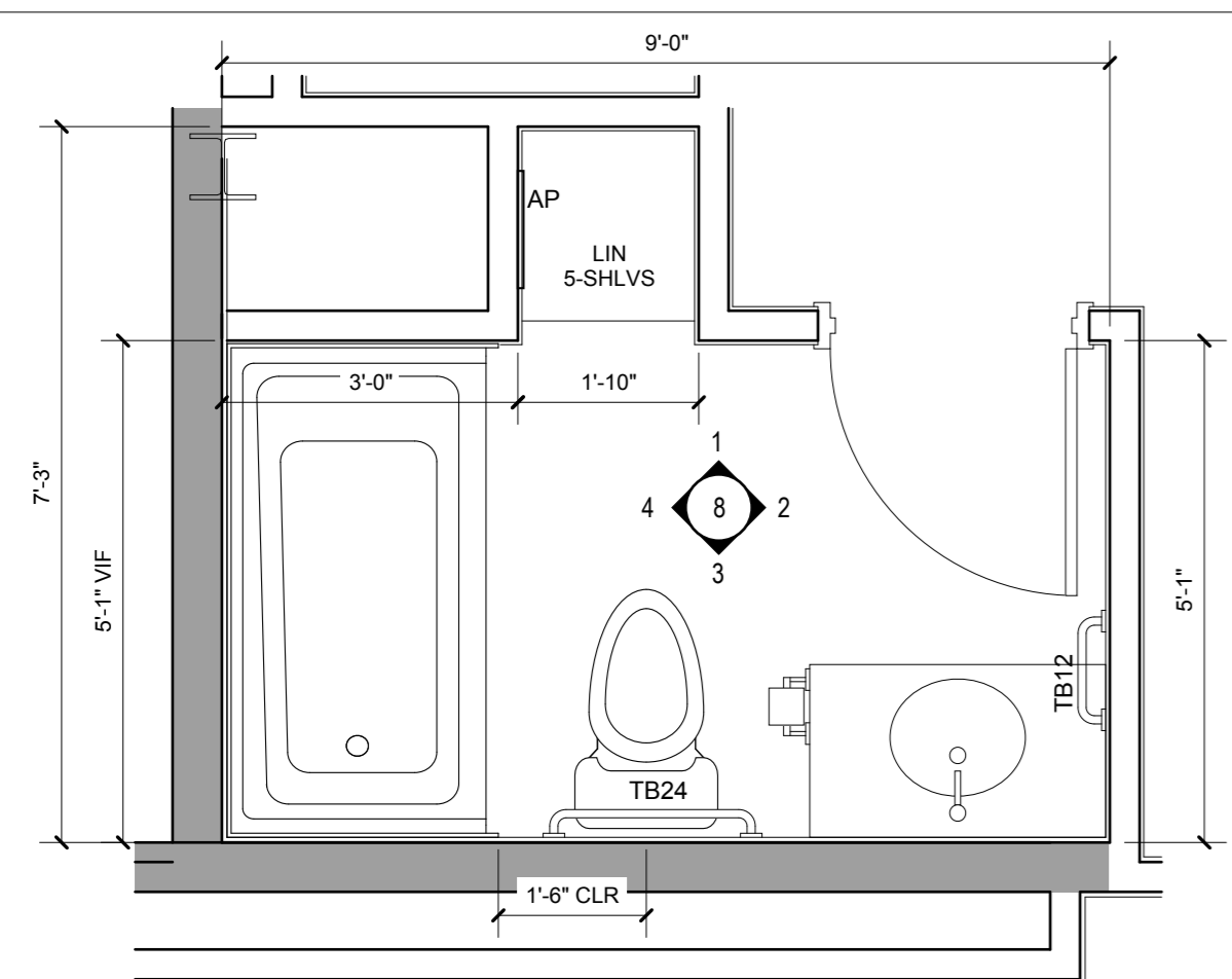
8 BATHROOM TYPE "H" SCALE: 1/2" = 1'-0"
