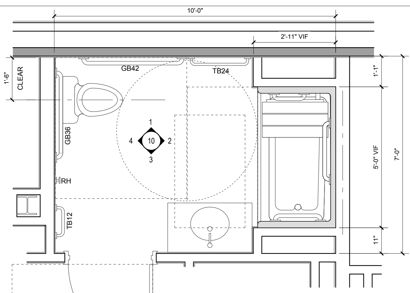
10 BATHROOM TYPE "K" SCALE: 1/2" = 1'-0"
