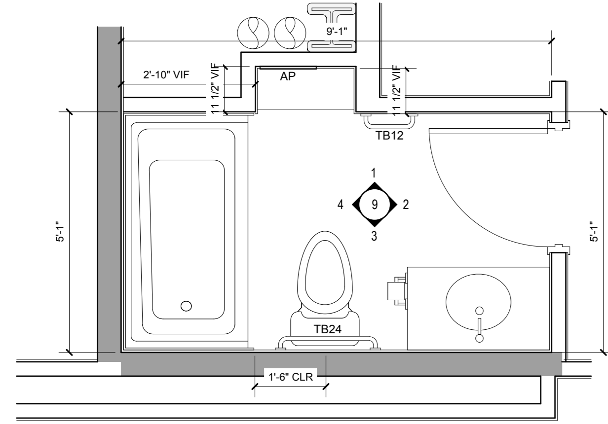
9 BATHROOM TYPE "J" SCALE: 1/2" = 1'-0"
