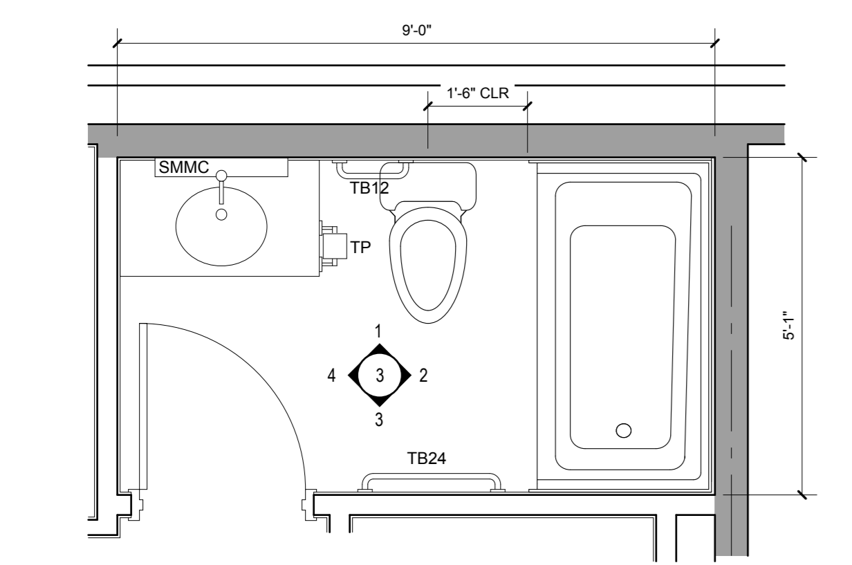
2 BATHROOM TYPE "B" SCALE: 1/2" = 1'-0"
