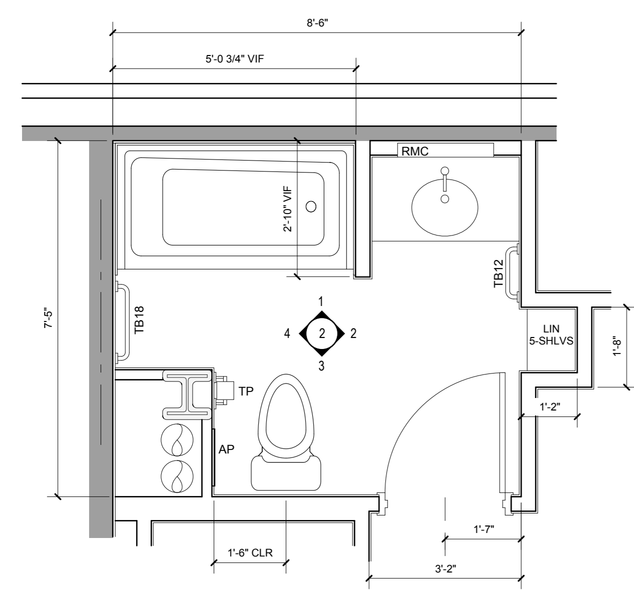
2 BATHROOM TYPE "B" SCALE: 1/2" = 1'-0"
