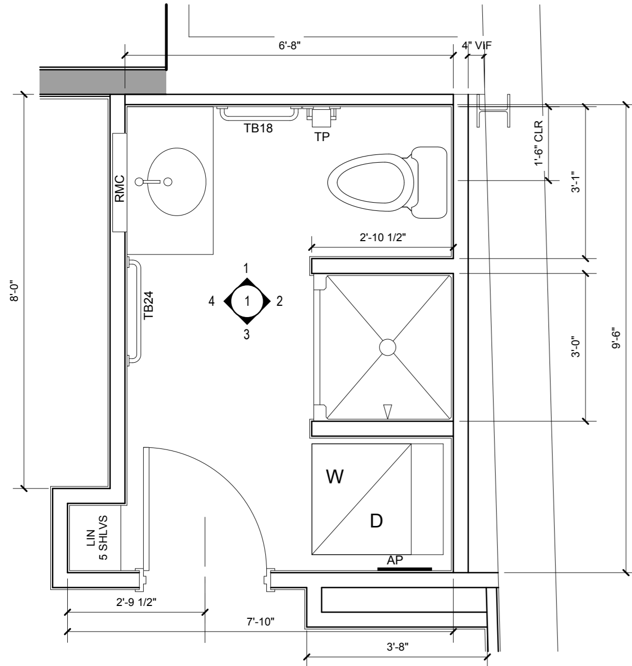
1 BATHROOM TYPE "A" SCALE: 1/2" = 1'-0"
