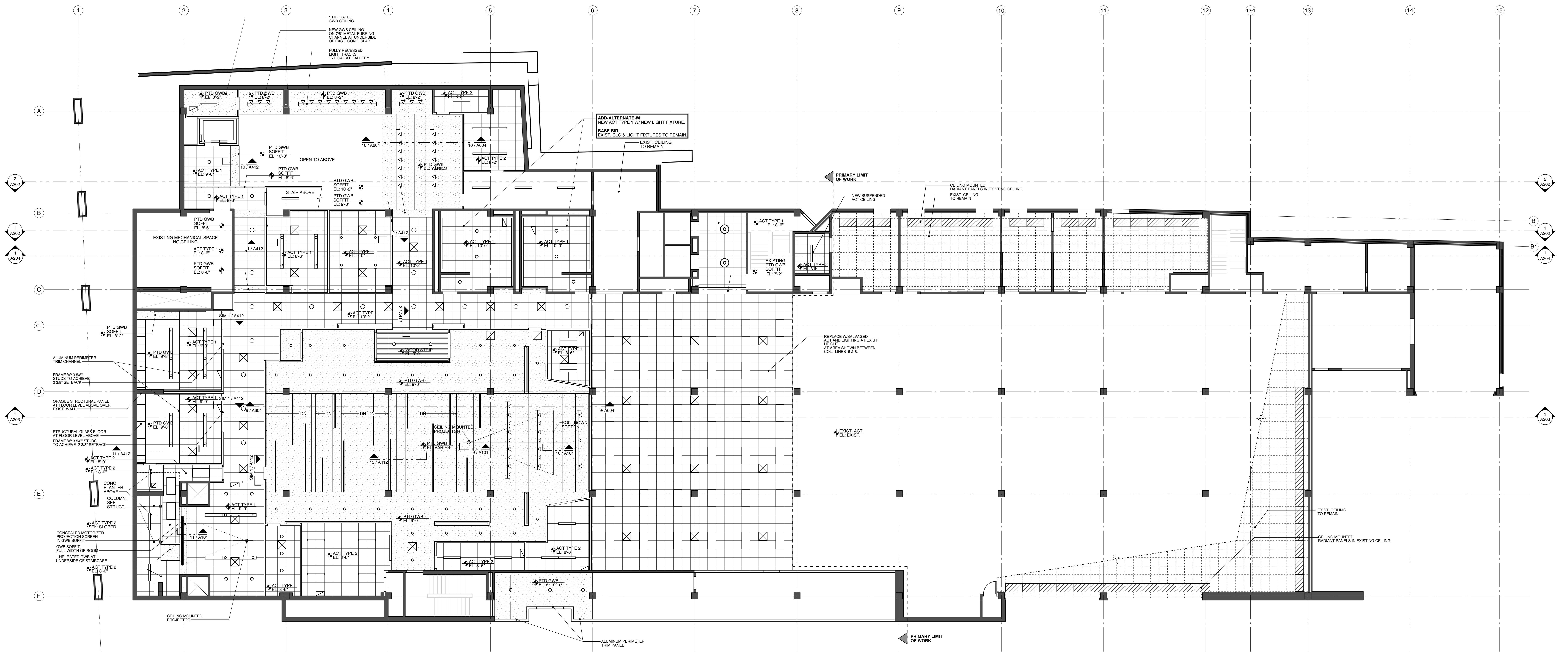
1 LOWER LEVEL RCP SCALE: 1/8" = 1'-0"
