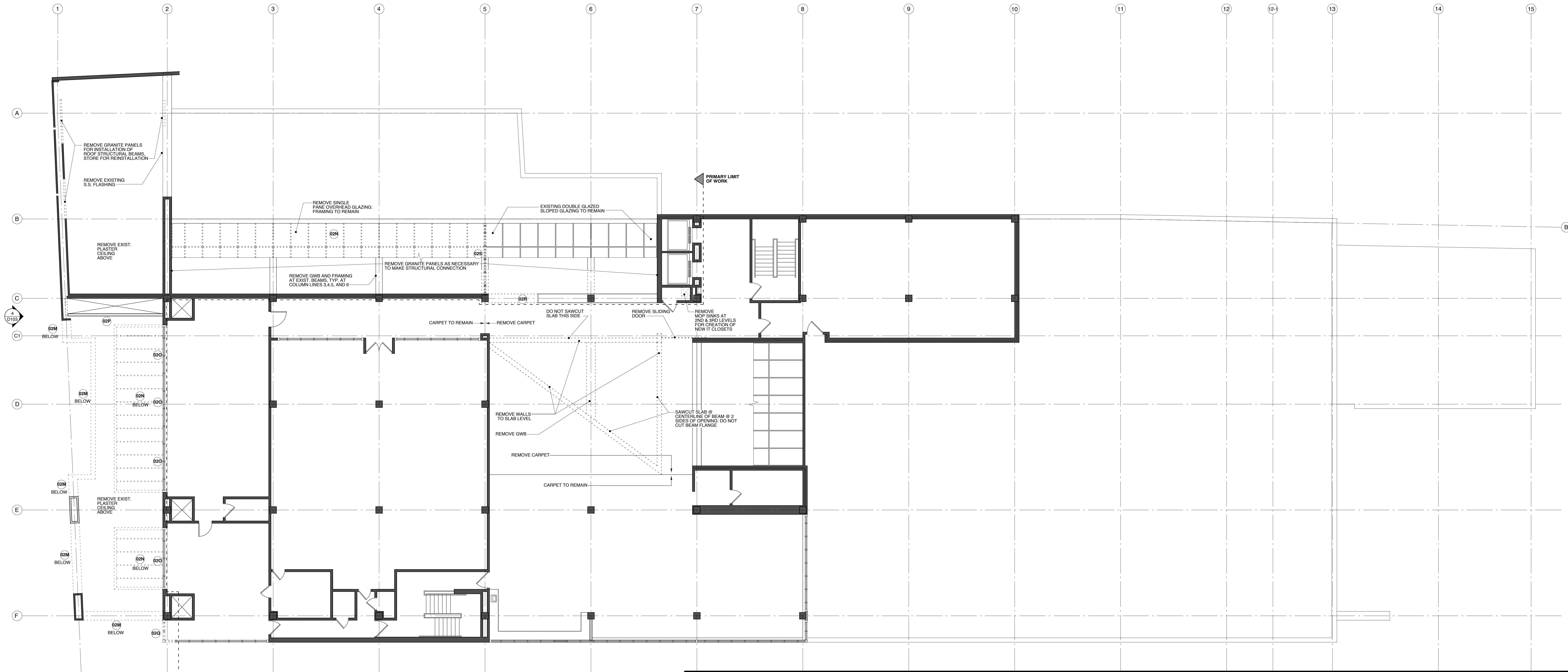
1 LEVEL 2 DEMO PLAN SCALE: 1/8" = 1'-0"
