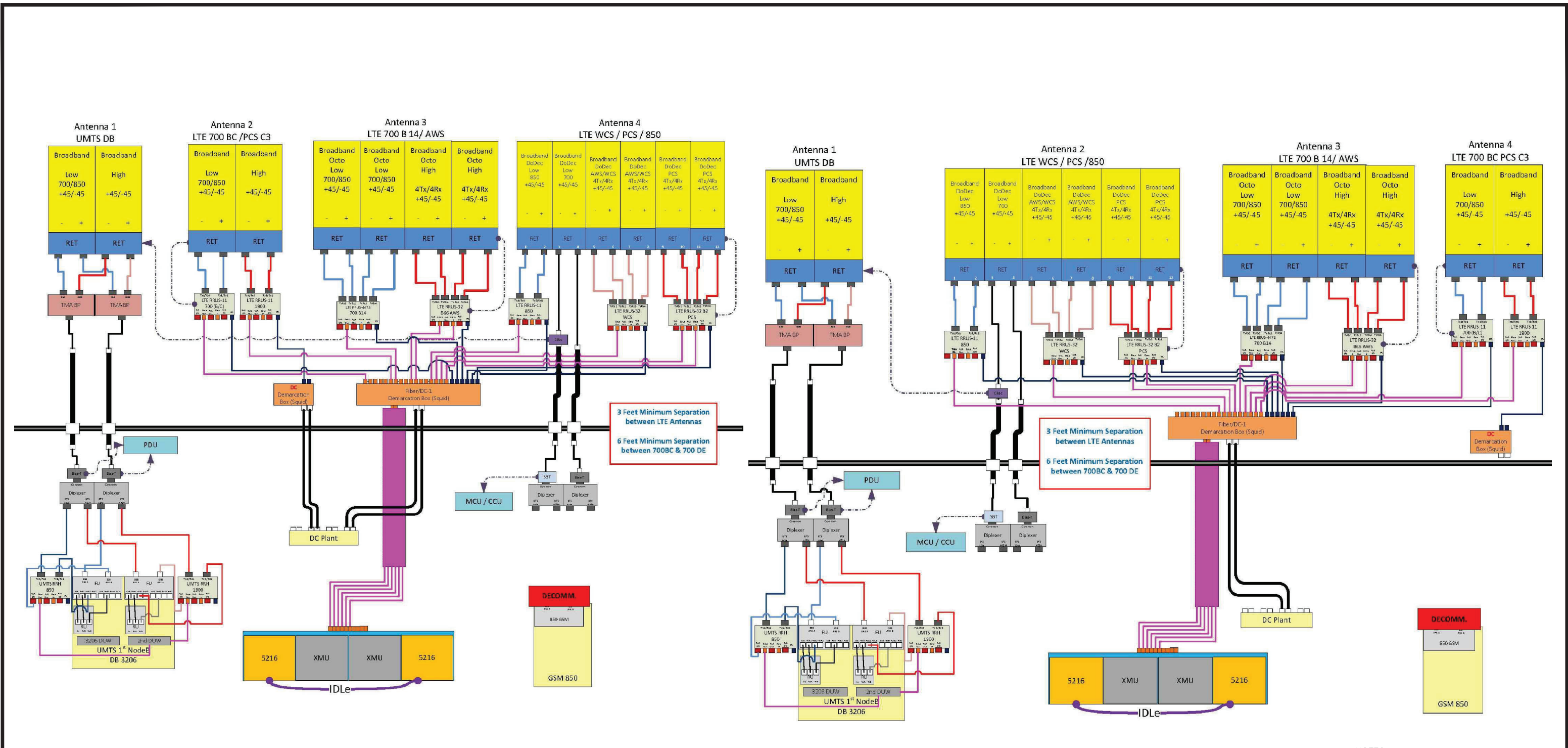
RF PLUMBING DIAGRAM ALPHA & BETA SECTOR SCALE: N.T.S. 1 RF-1
