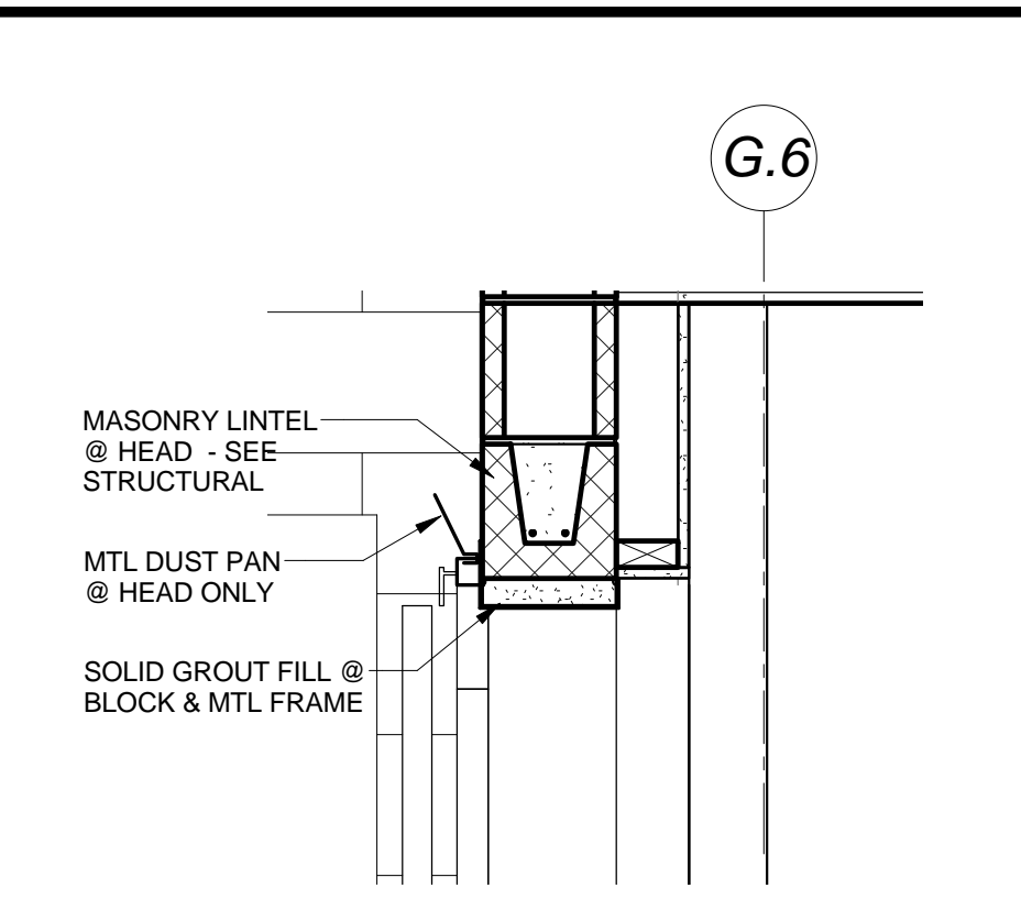
E3 ELEVATOR DOOR HEAD DETL (JAMB SIMILAR) 1" = 1'-0"
