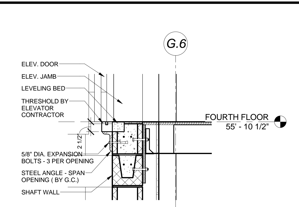
E2 ELEVATOR DOOR BASE DETAIL 1" = 1'-0"
