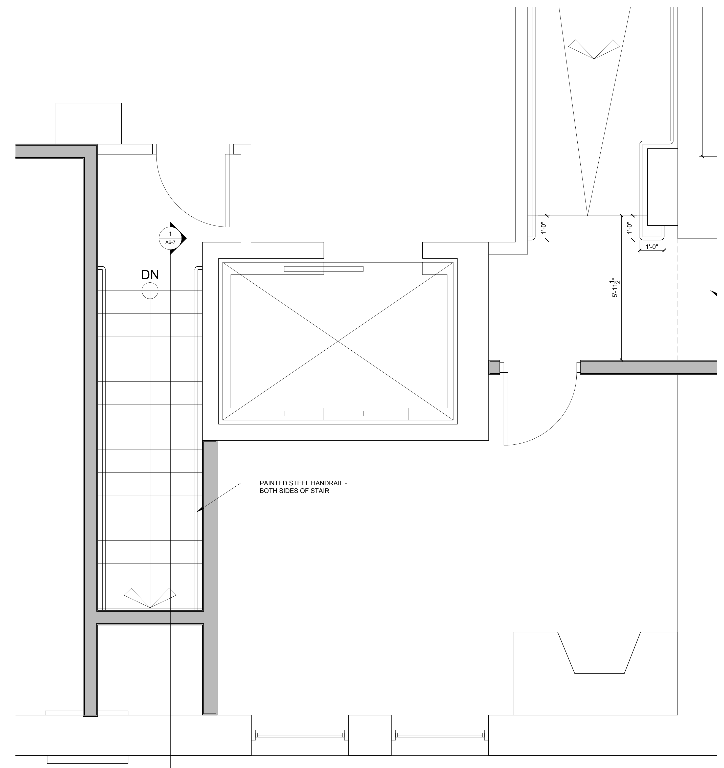
1 STAIR ONE (200) 1/2\"/>
