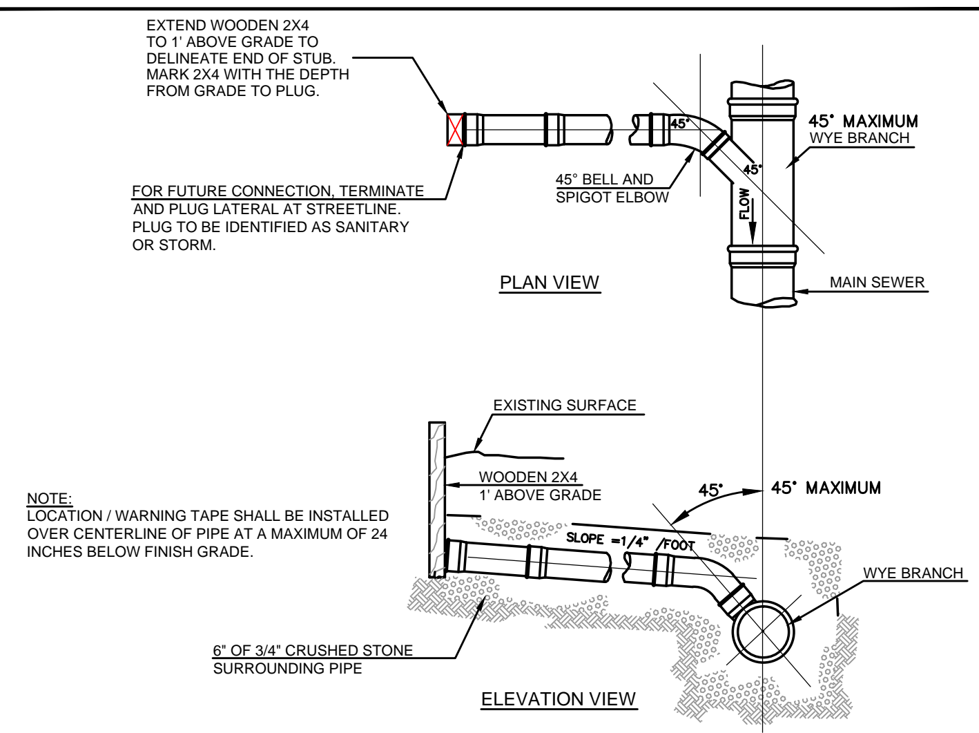
(D) TYPICAL LATERAL TEE/WYE CONNECTION N.T.S.
