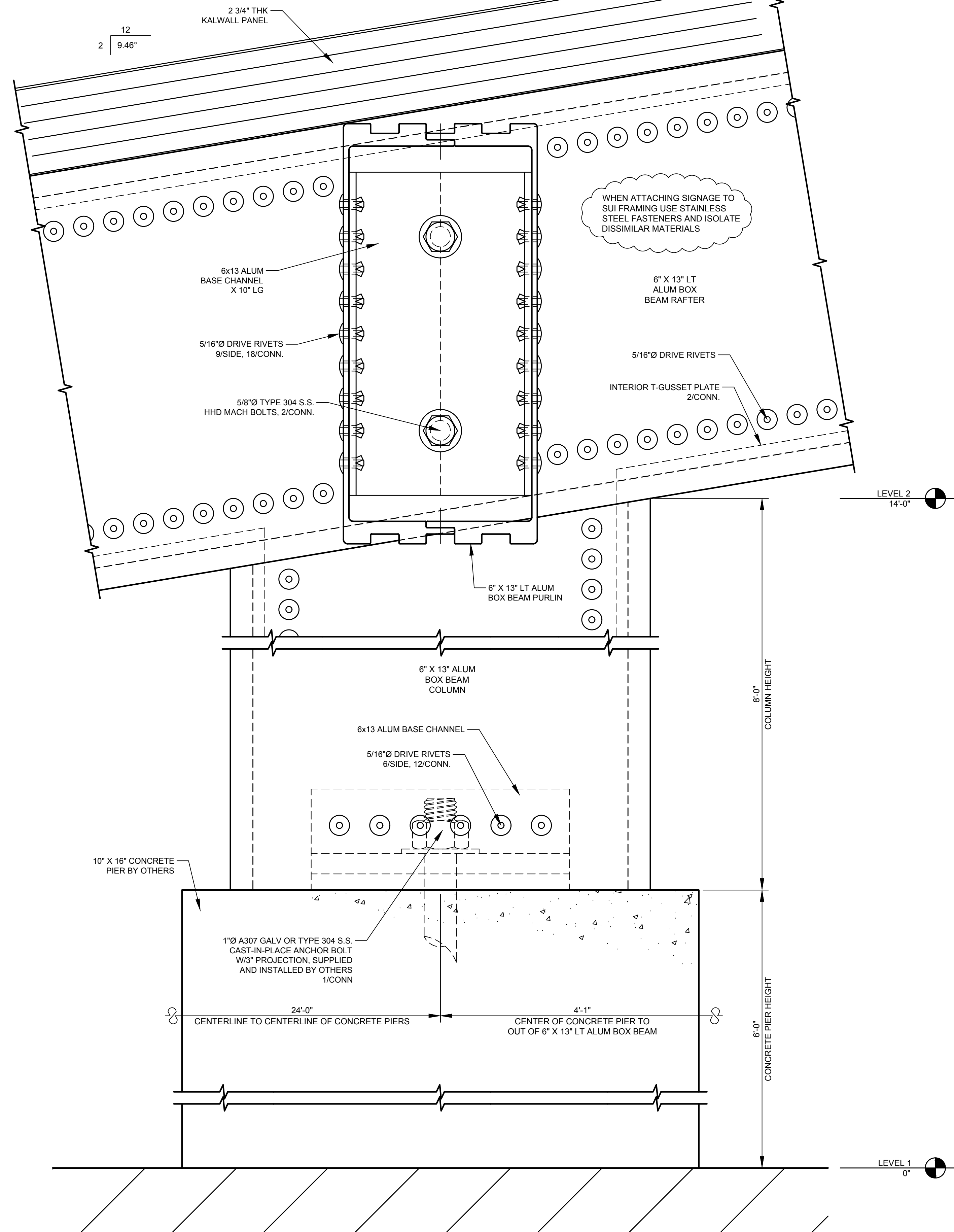
SECTION 2 SCALE: 1/2" = 1'
