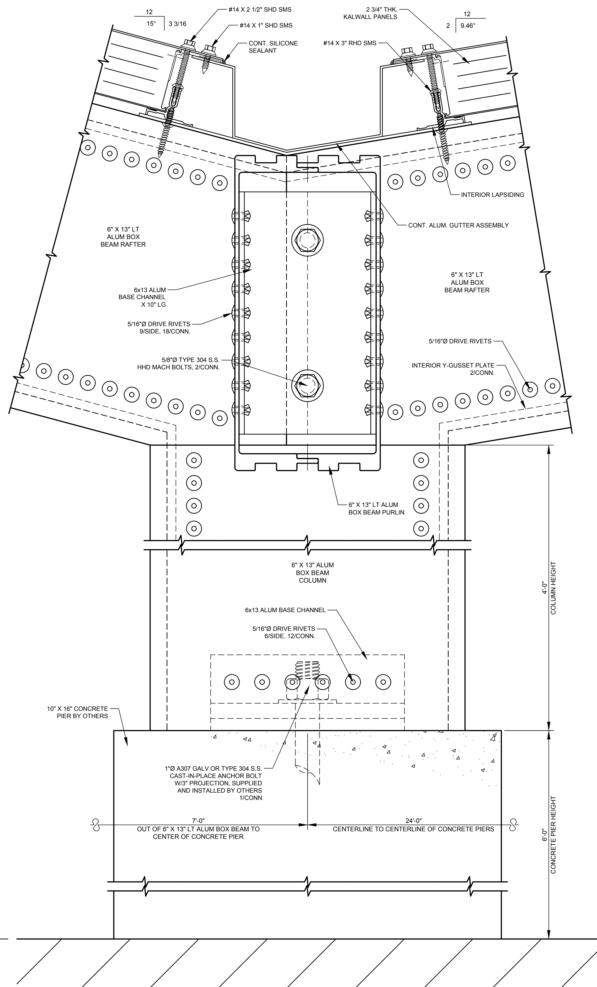
SECTION 1 SCALE: 1/2" = 1'
