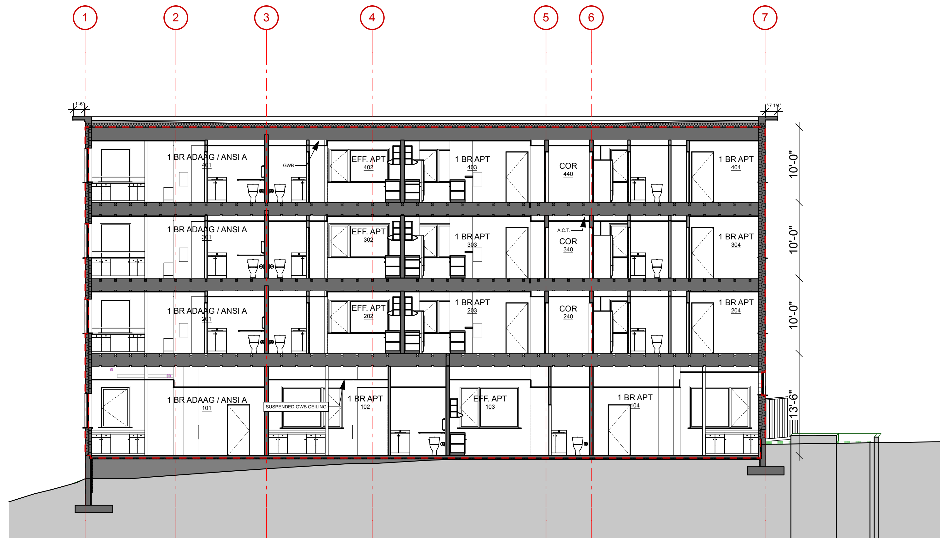
2 SECTION: E/W SCALE: 1/8" = 1'-0"
