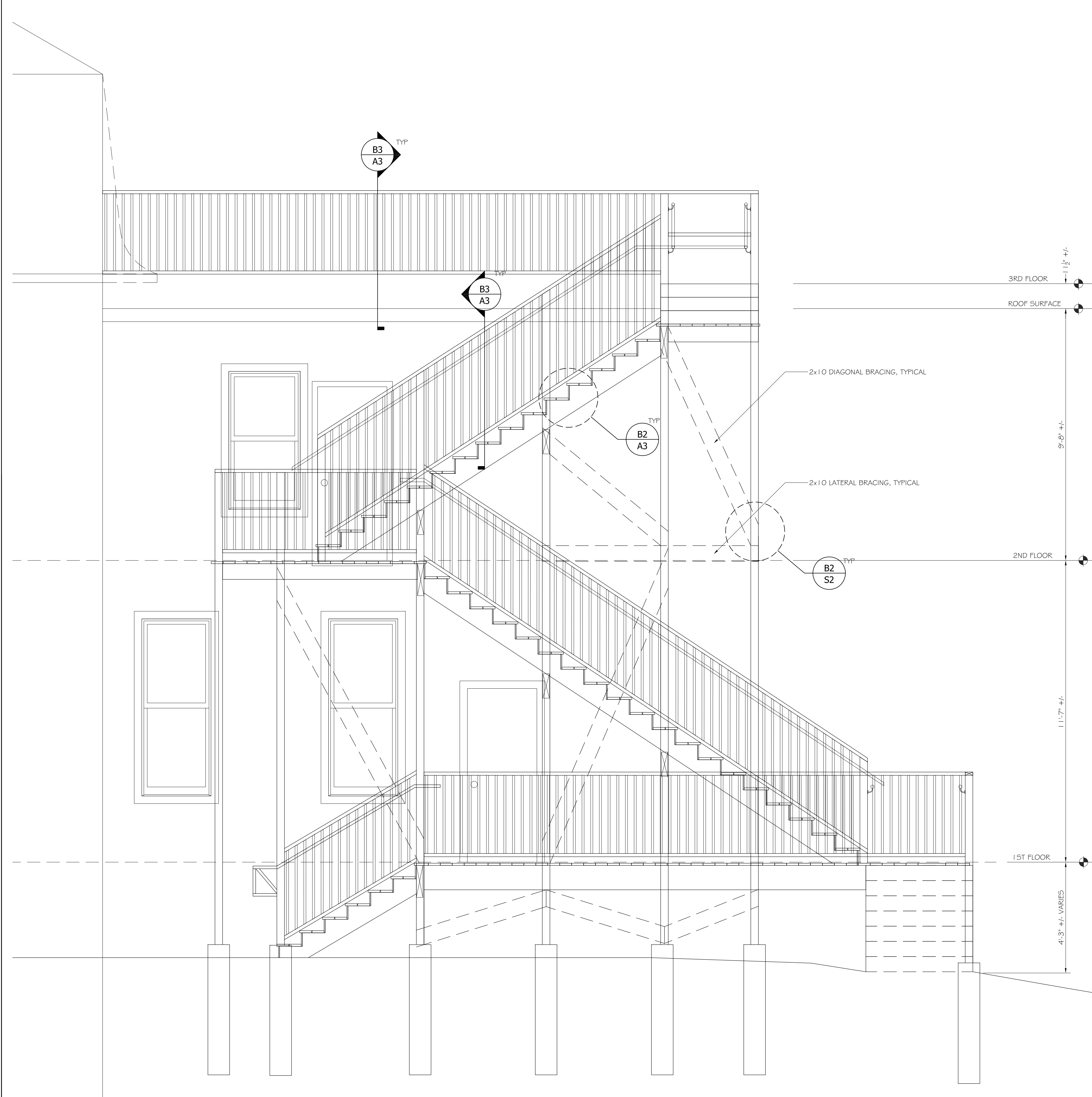
A1 STAIR ELEVATION - SIDE SCALE: 1/2" = 1'-0"
