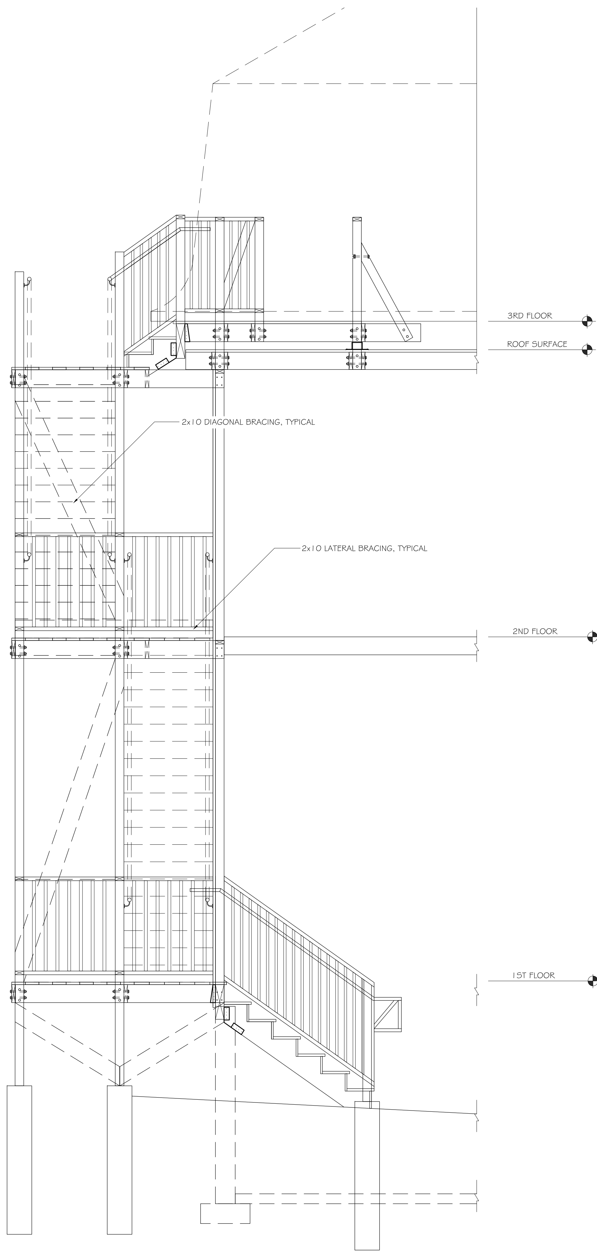
A3 STAIR ELEVATION - REAR SCALE: 1/2" = 1'-0"
