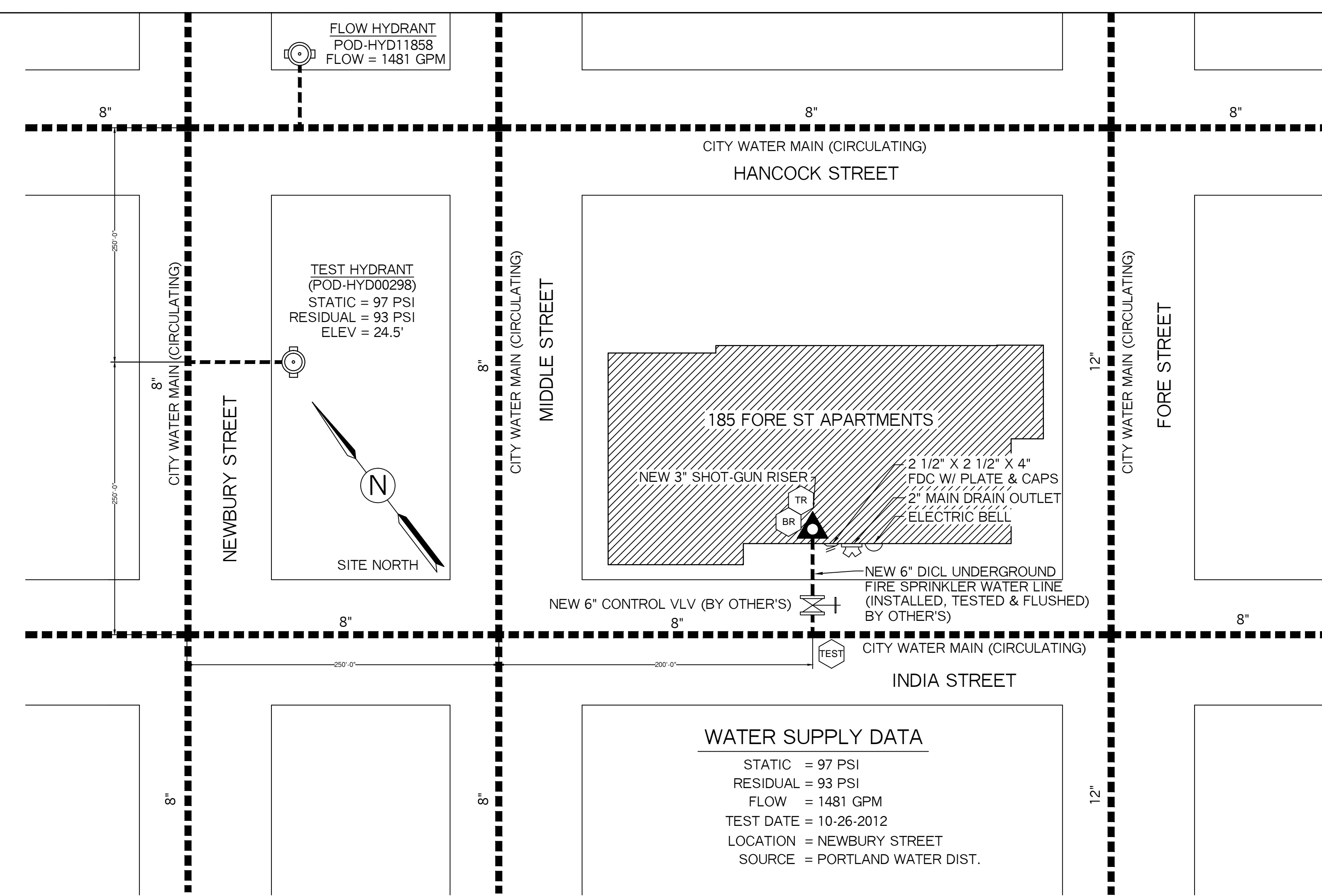
PLOT / SITE PLAN N.T.S.
