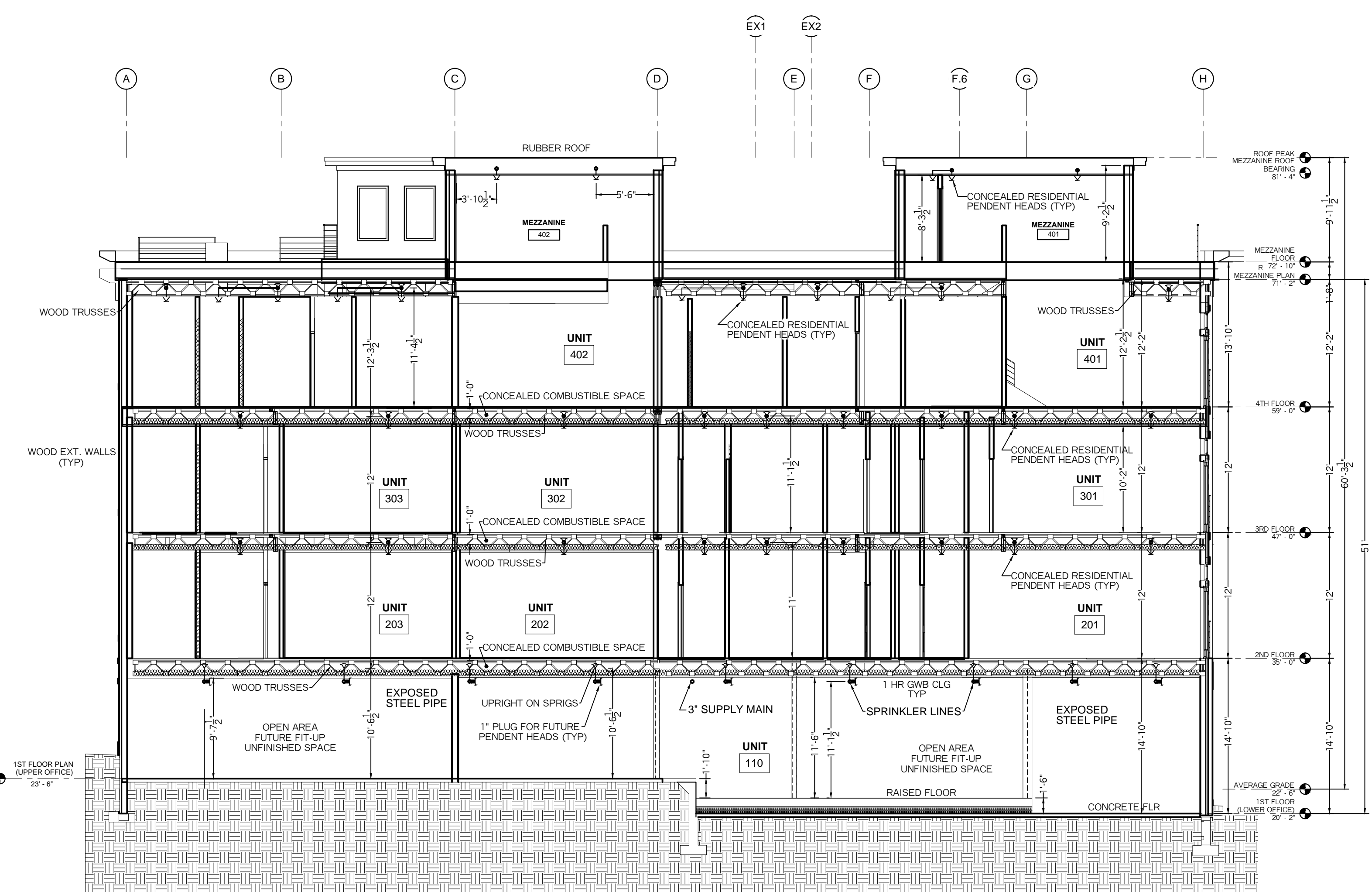
BUILDING SECTION A-A SCALE: 1/8" = 1'-0"
