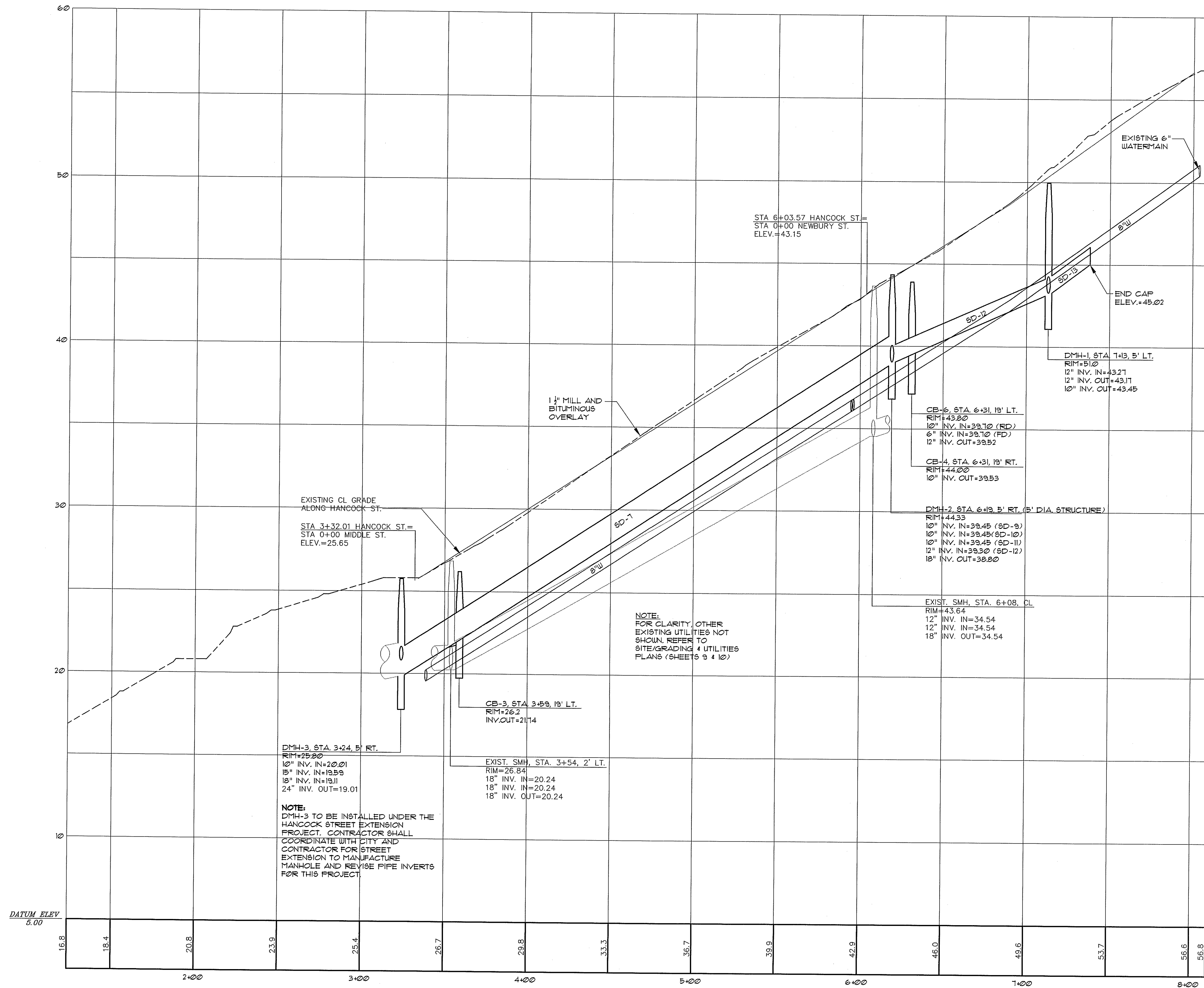
PROFILE: HANCOCK STREET HORIZ. SCALE: 1" = 30' VERT. SCALE: 1" = 3'
