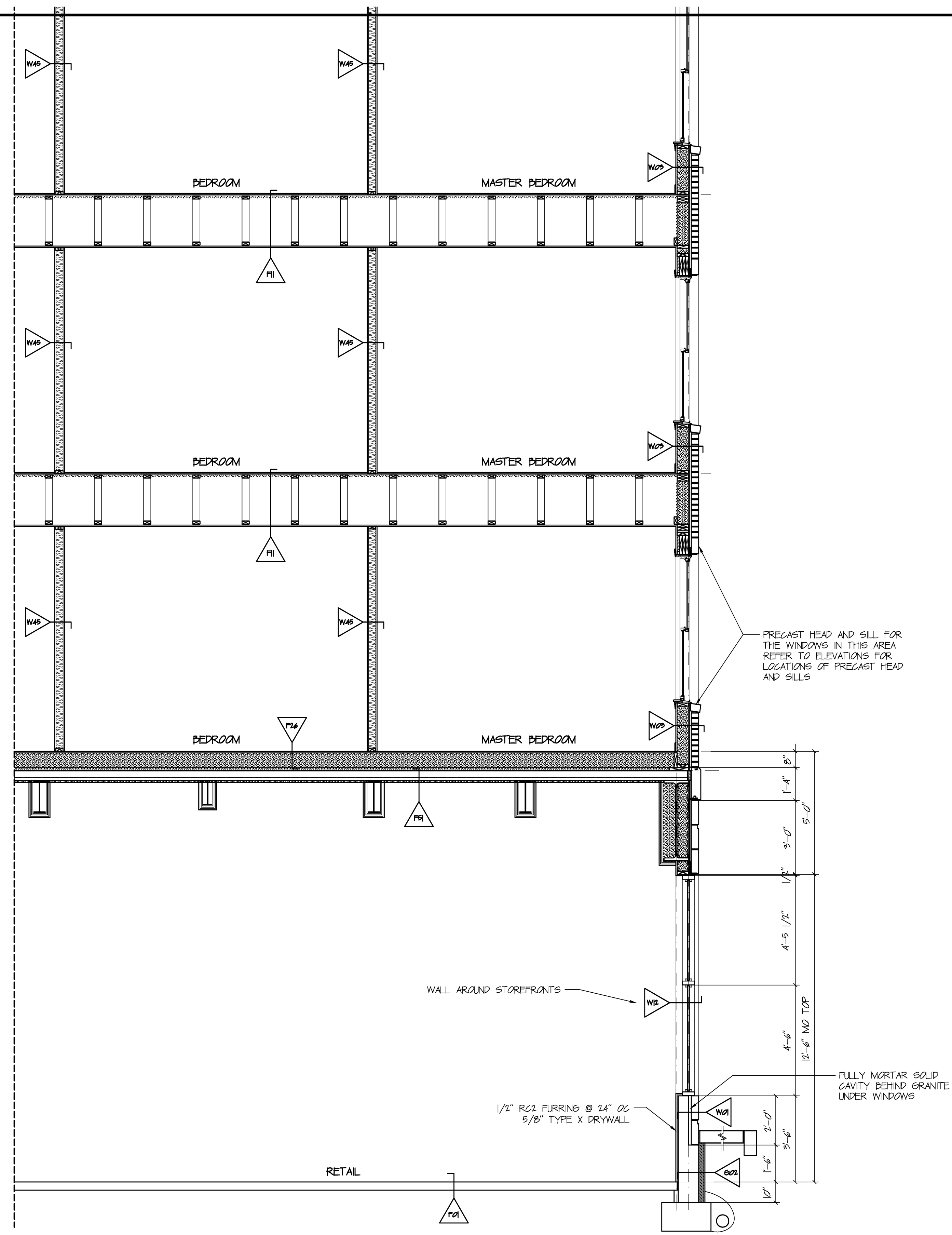
SECTION 07 SCALE: 3/8" = 1' 0"
