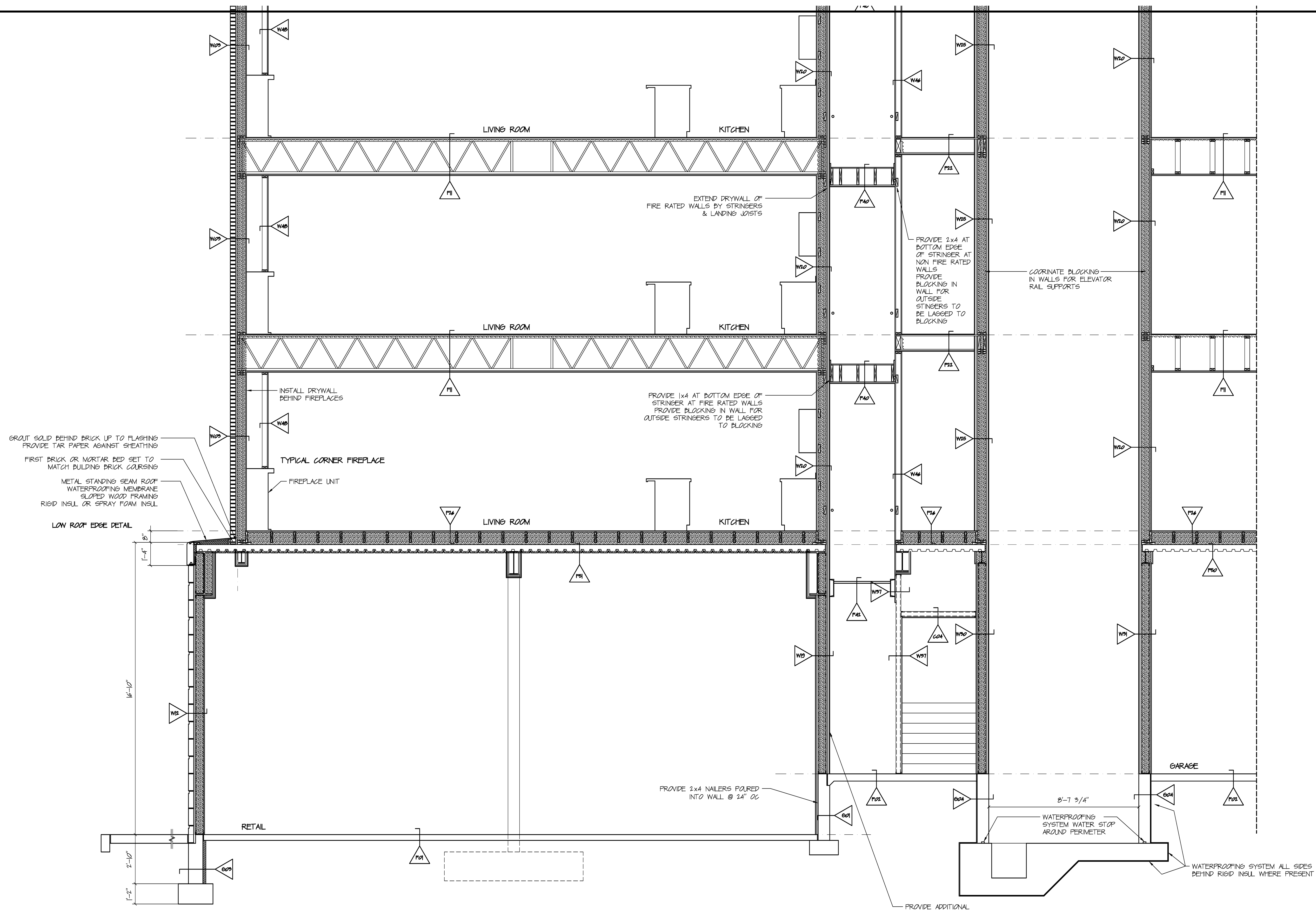
SECTION 04 SCALE: 3/8" = 1' 0"
