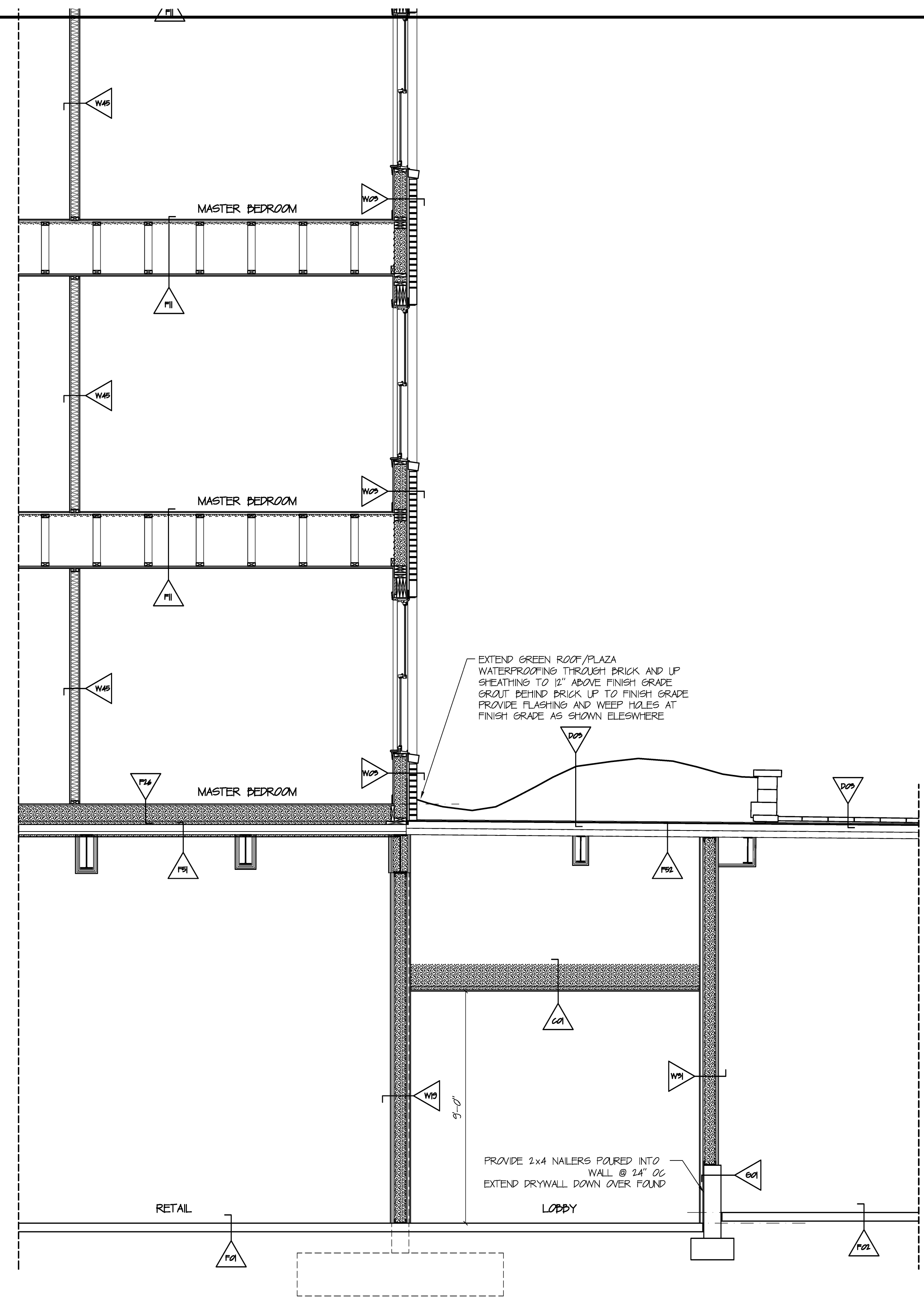
SECTION 35 SCALE: 3/8" = 1' 0"
