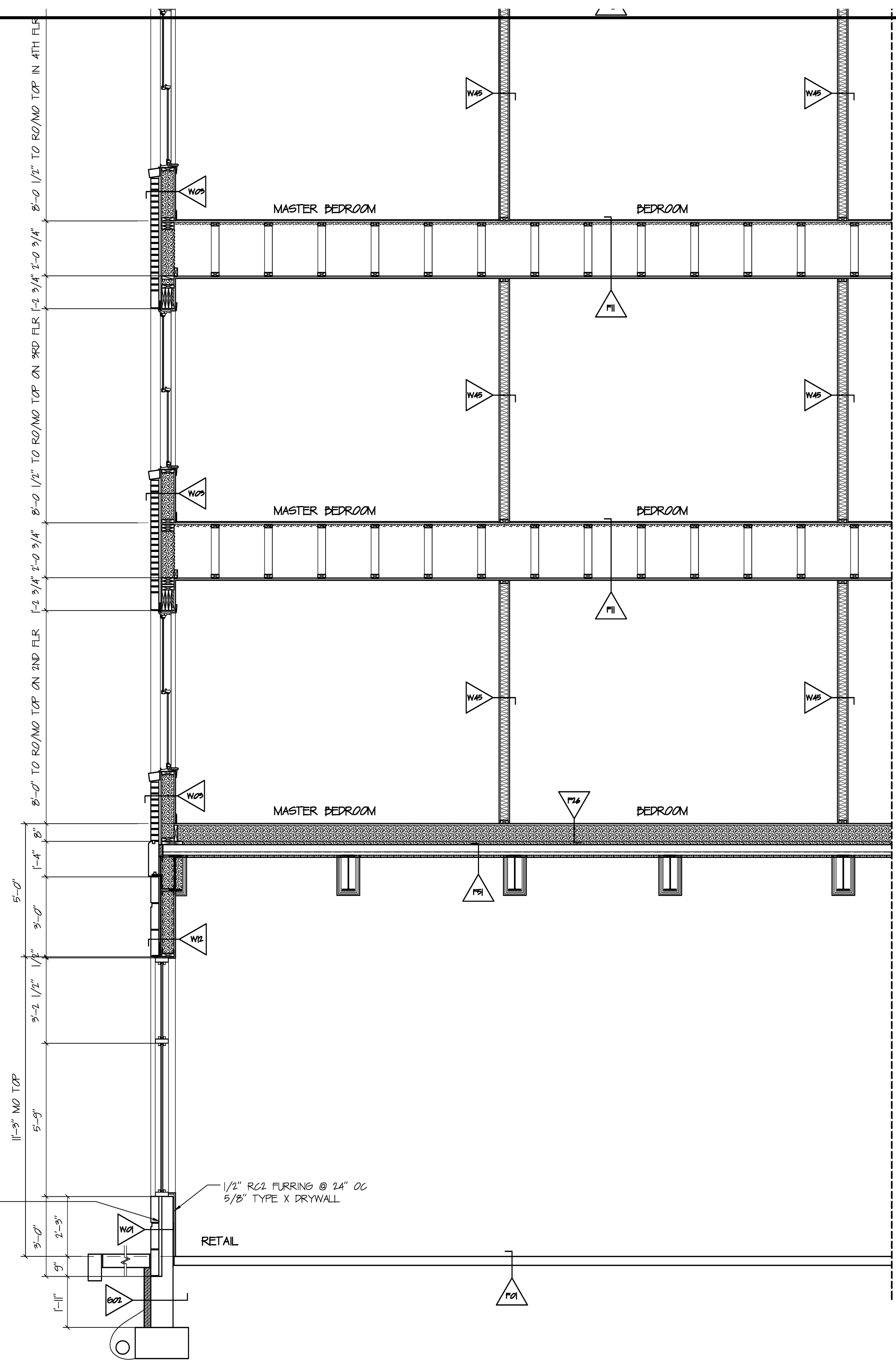
SECTION 22 SCALE: 3/8" = 1' 0"
