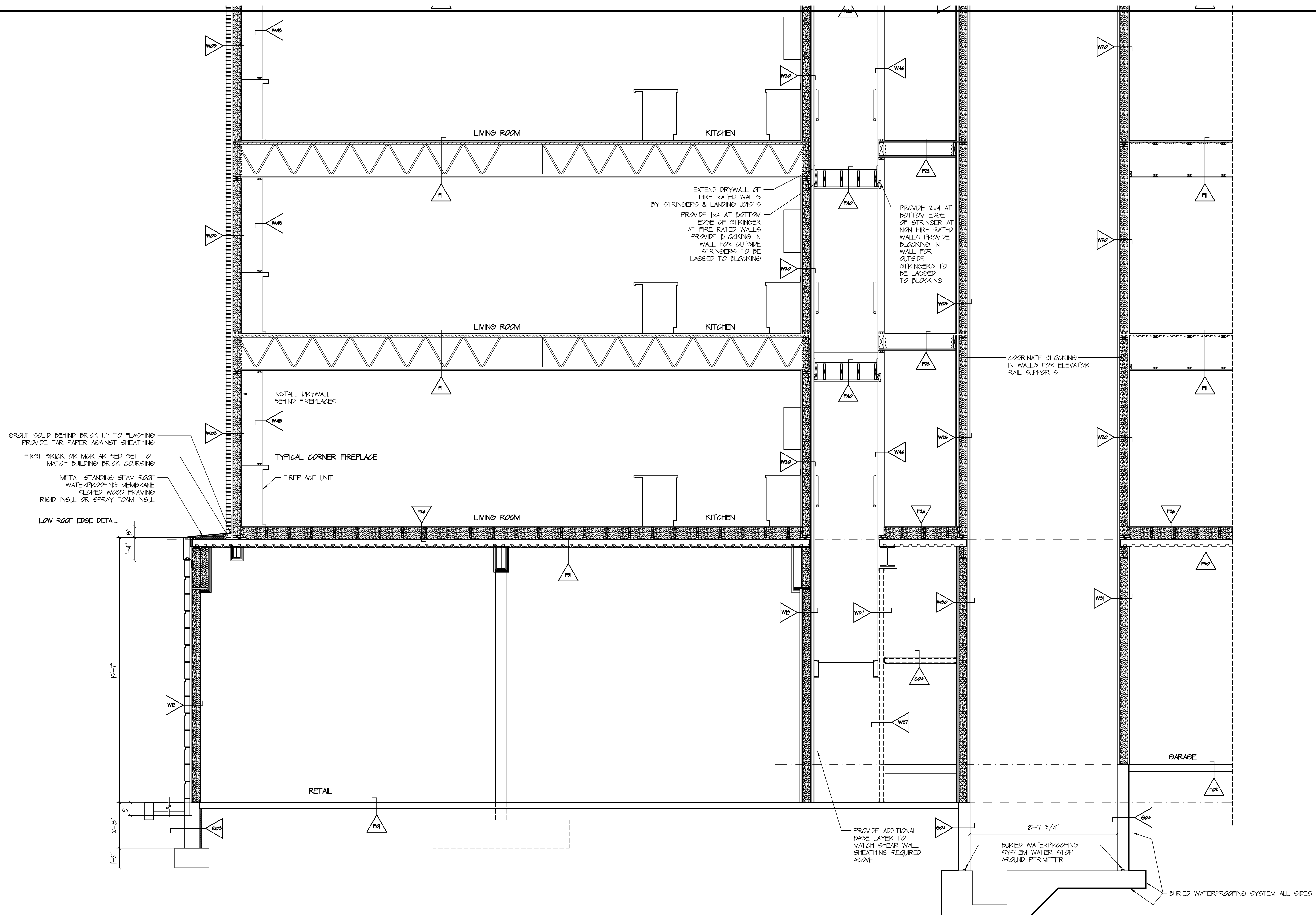
SECTION 18 SCALE: 3/8" = 1' 0"
