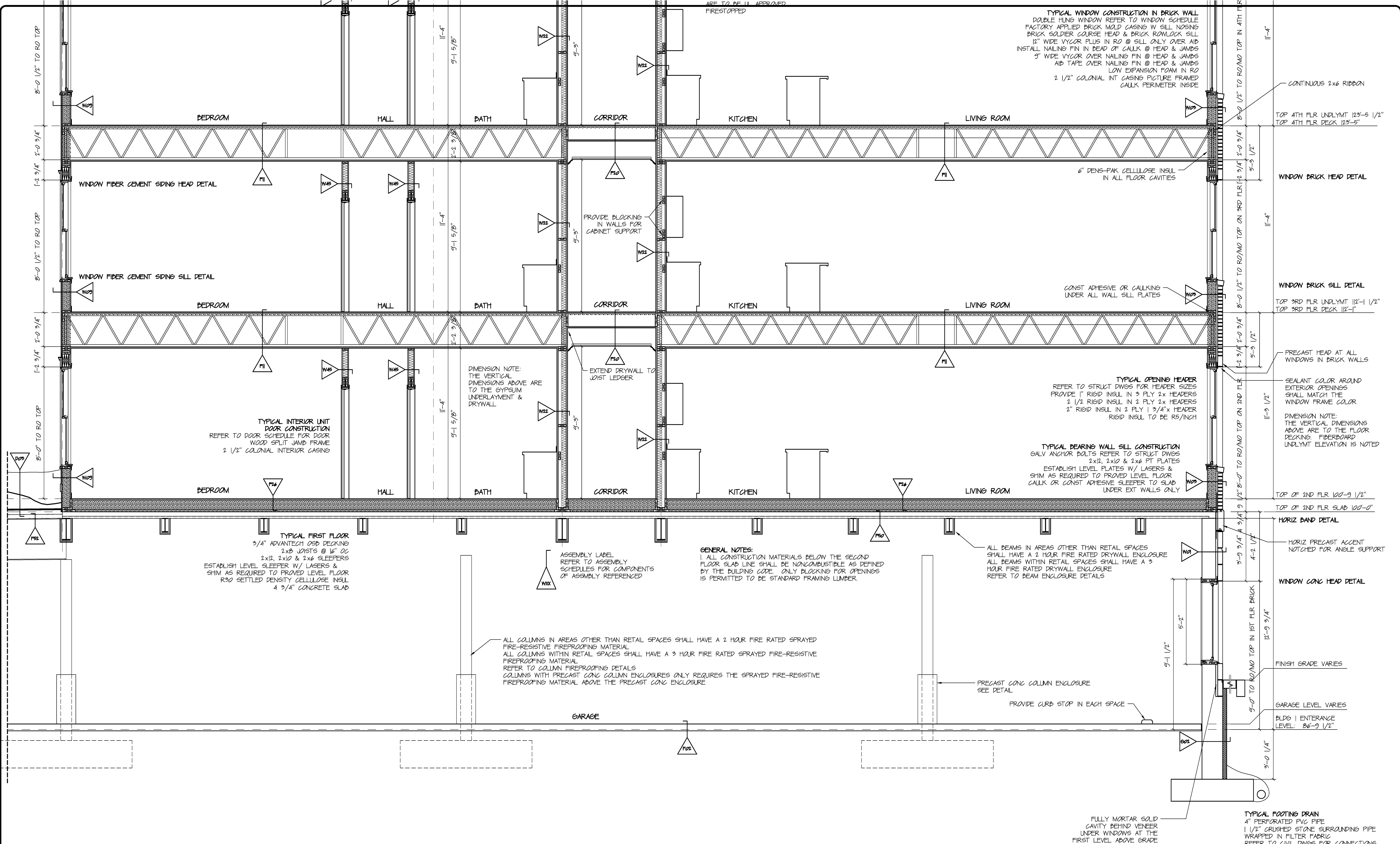
SECTION 01 SCALE: 3/8" = 1' 0"
