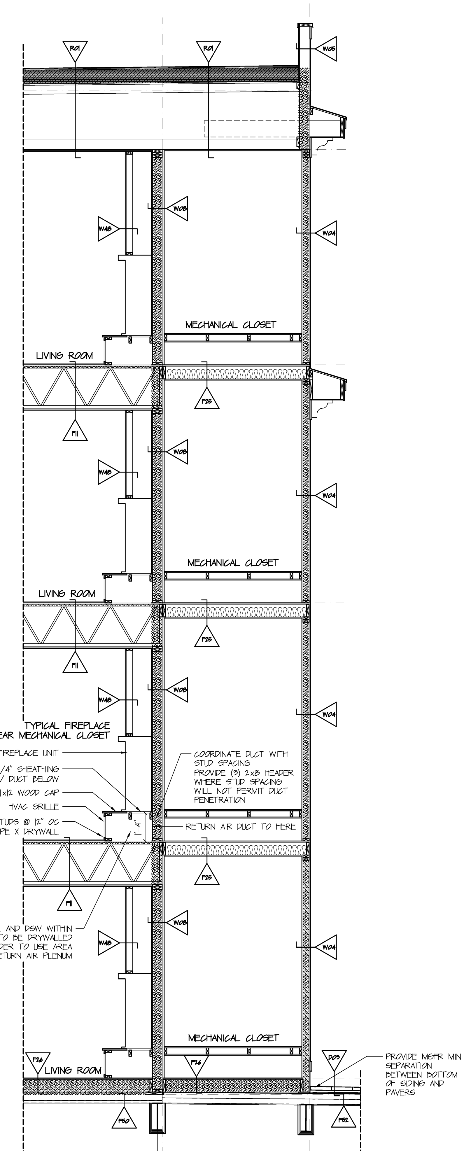
SECTION P SCALE: 3/8" = 1' 0"
