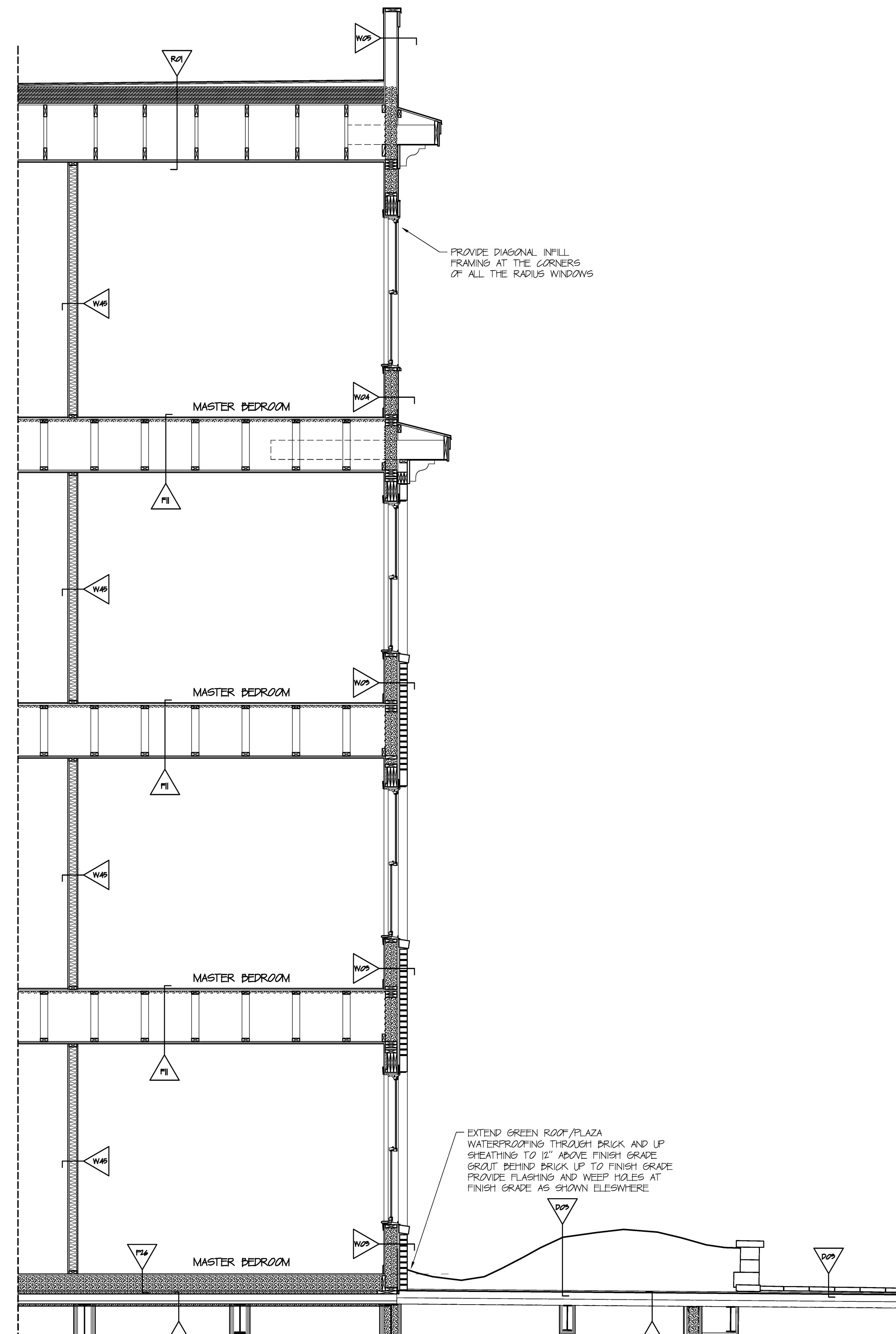
SECTION Y SCALE: 3/8" = 1' 0"
