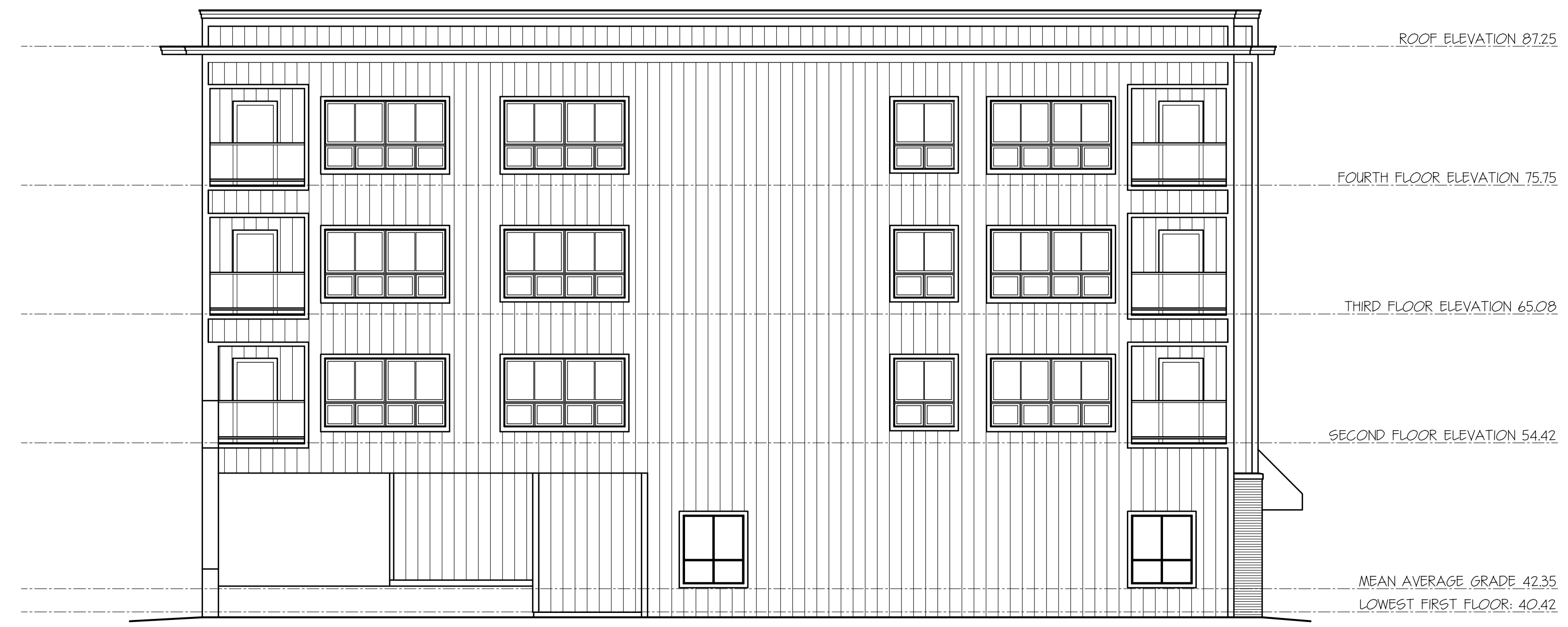
LEFT SIDE ELEVATION SCALE: 1/8" = 1' 0"
